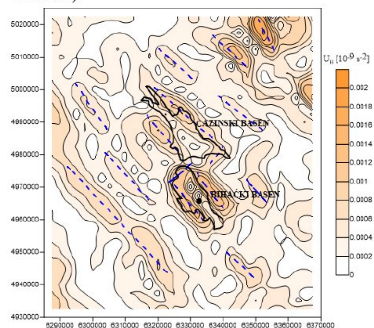
Slika 5 – Karta ukupnog horizontalnog gradijenta sa prikazanim položajem Bihačkog i Cazinskog bazena (plave isprekidane linije-interpretirani kontakti)
