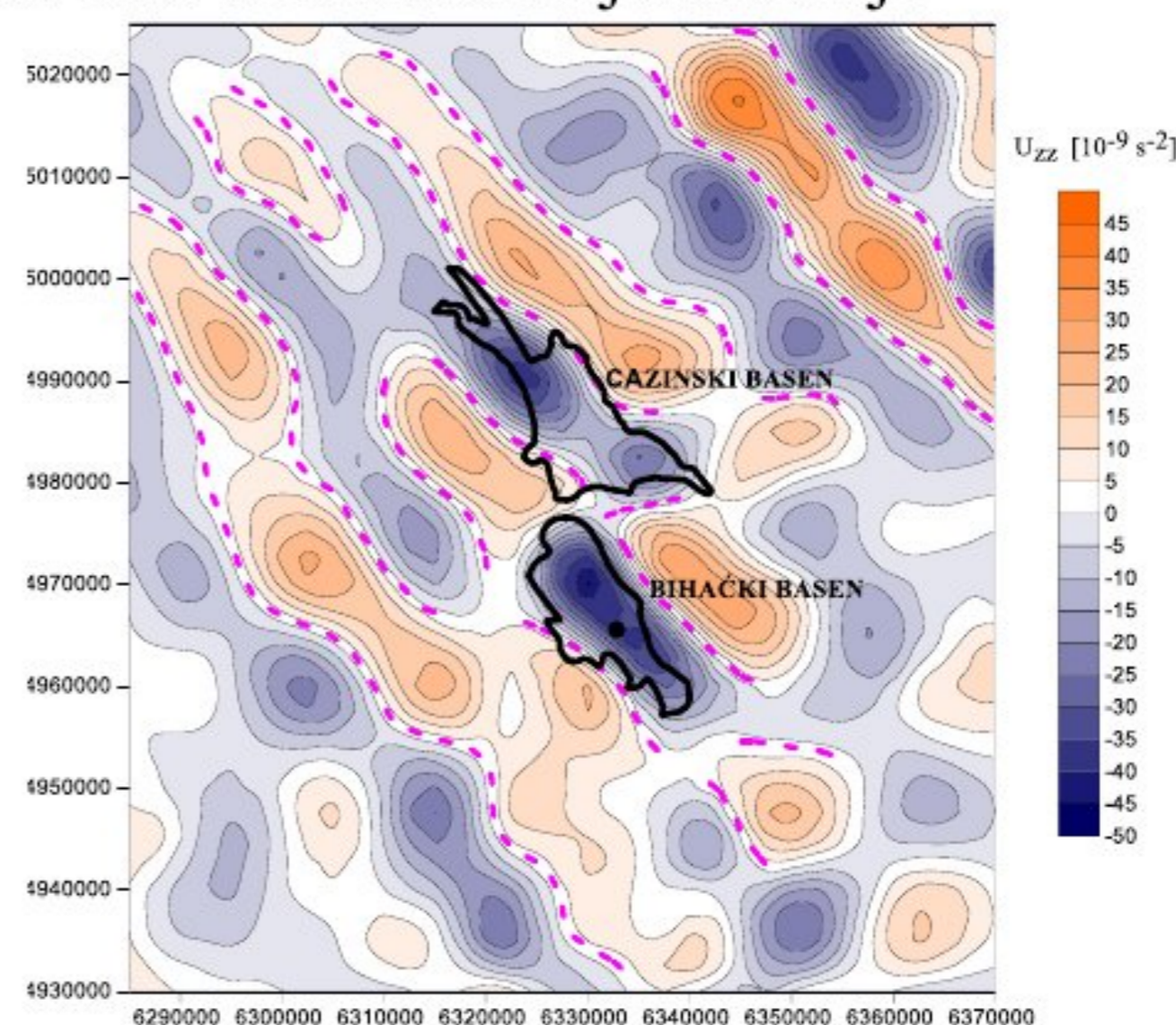
Slika 4 – Karta vertikalnog gradijenta sa prikazanim položajem Bihačkog i Cazinskog bazena (ljubičaste isprekidane linije-interpretirani kontakti)
