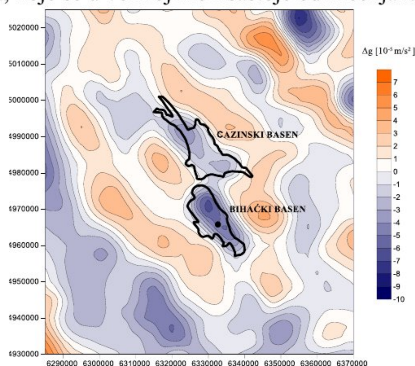
Slika 3 – Karta filtriranih lokalnih gravimetrijskih anomalija sa prikazanim položajem Bihačkog i Cazinskog bazena
