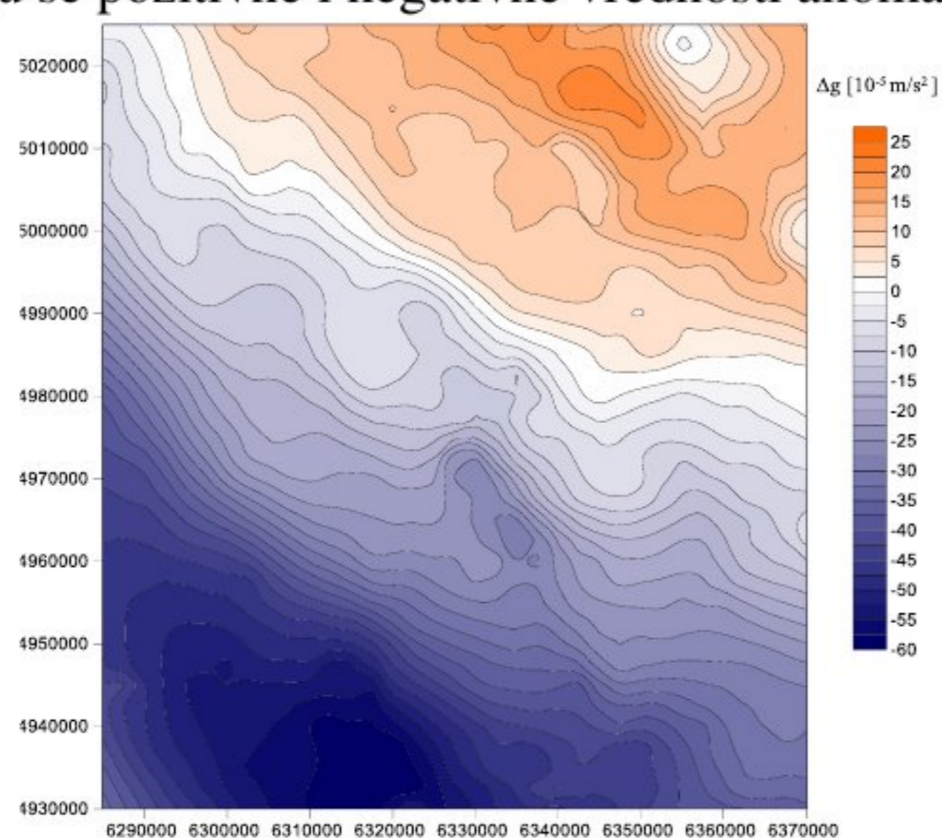
Slika 2 – Karta Bugeovih anomalija
