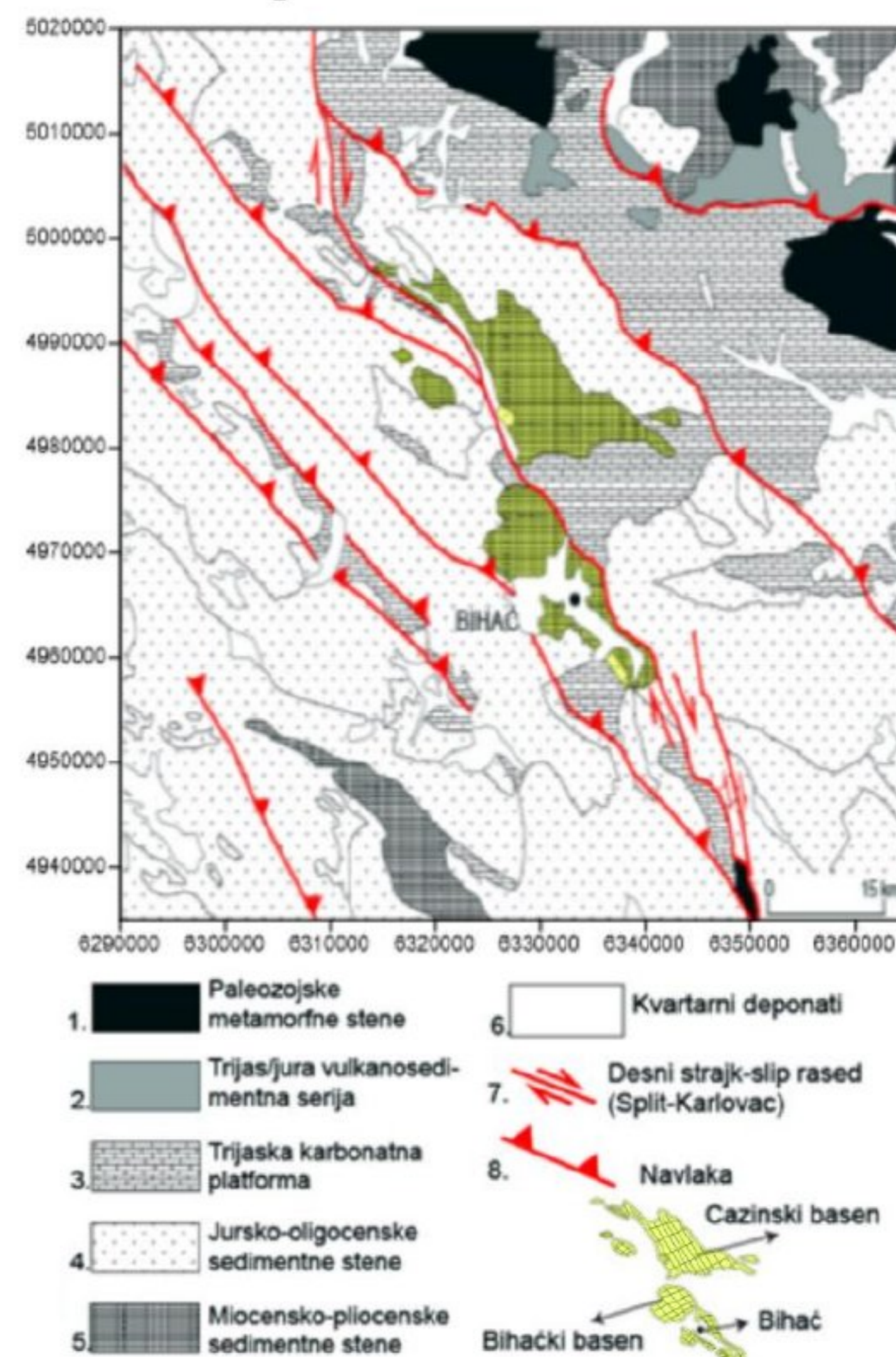
Slika 1 – Geološka karta istražnog terena (prema [6])
