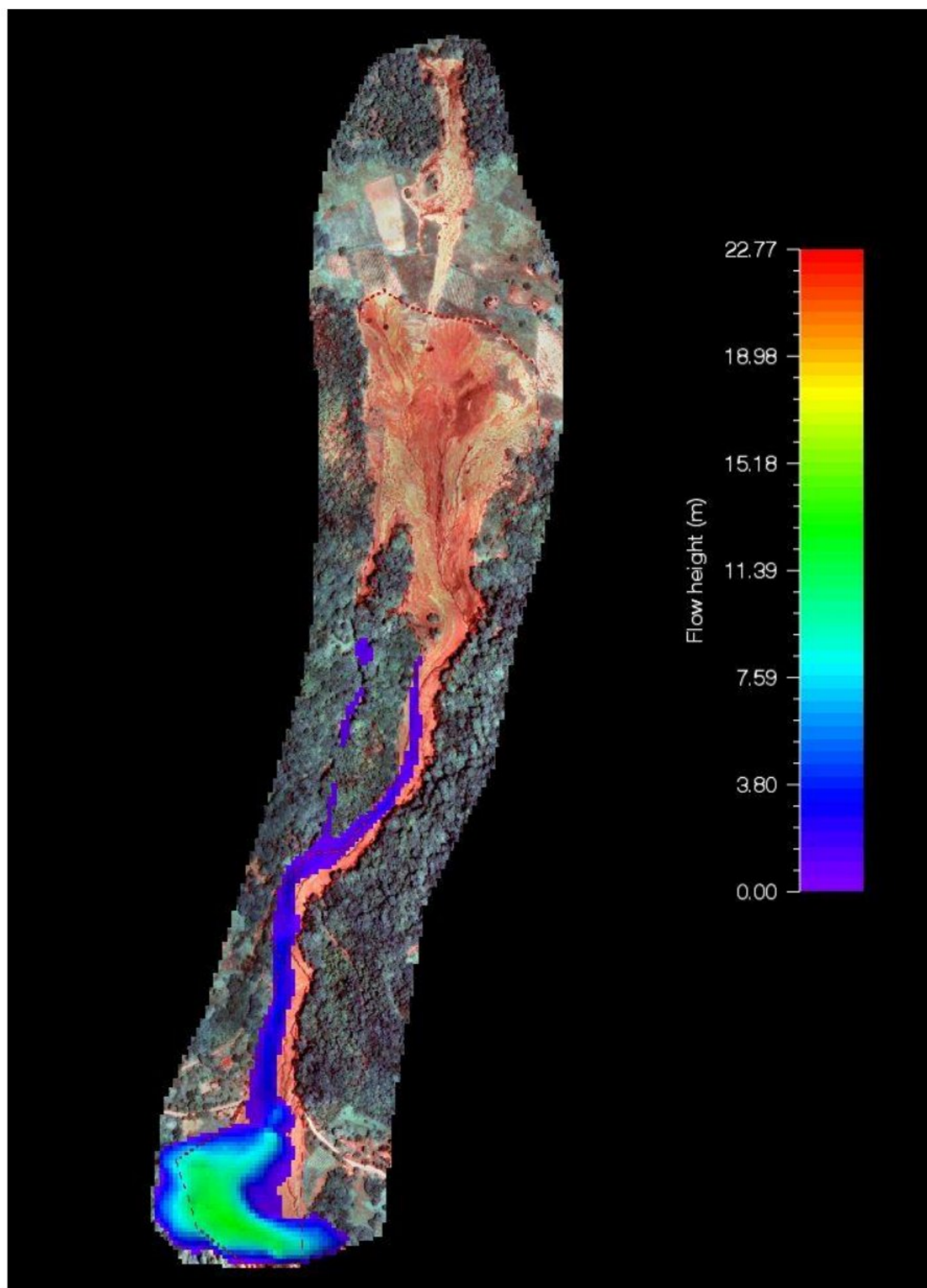
Слика 8.4 Модел финалних дубина тецишта Селанац на прецизнијем моделу терена са прорачуном приноса материјала (Krušič et. al., 2019)
