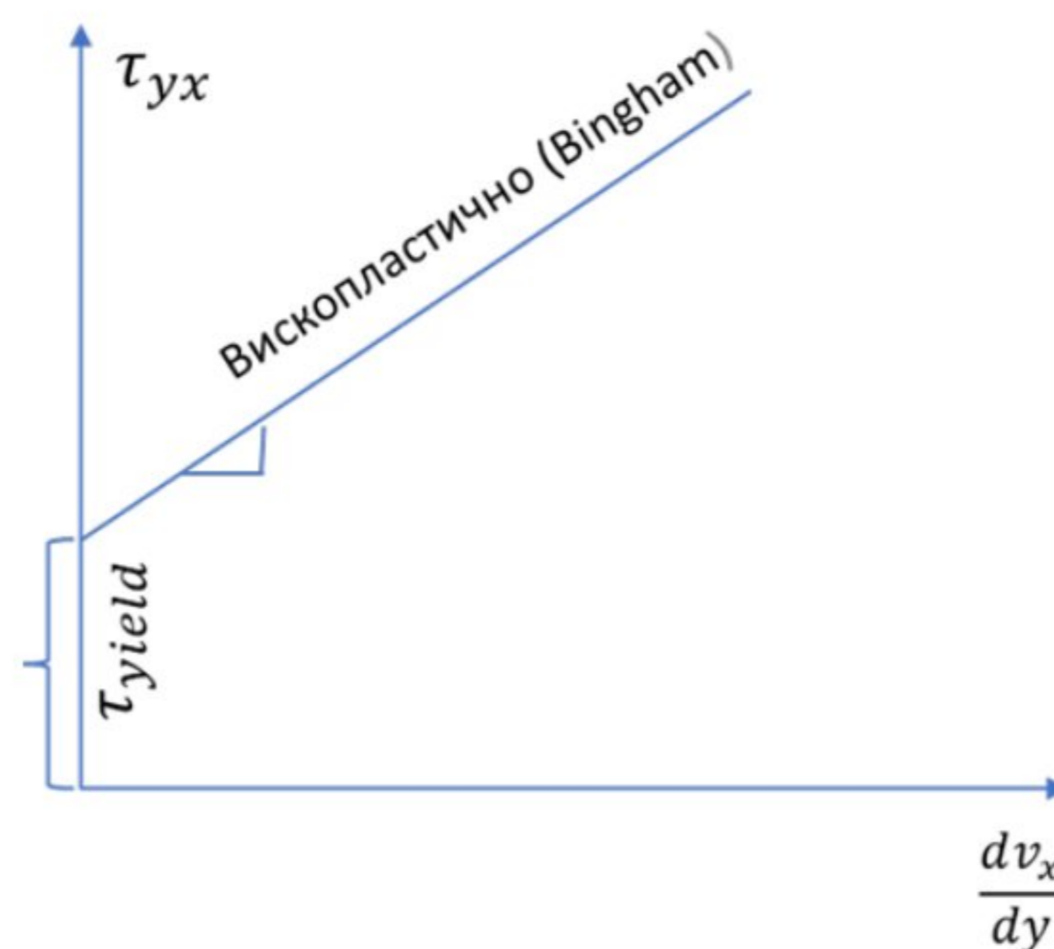
Слика 2.9 Бингамов (Bingham, 1922) критеријум течења
