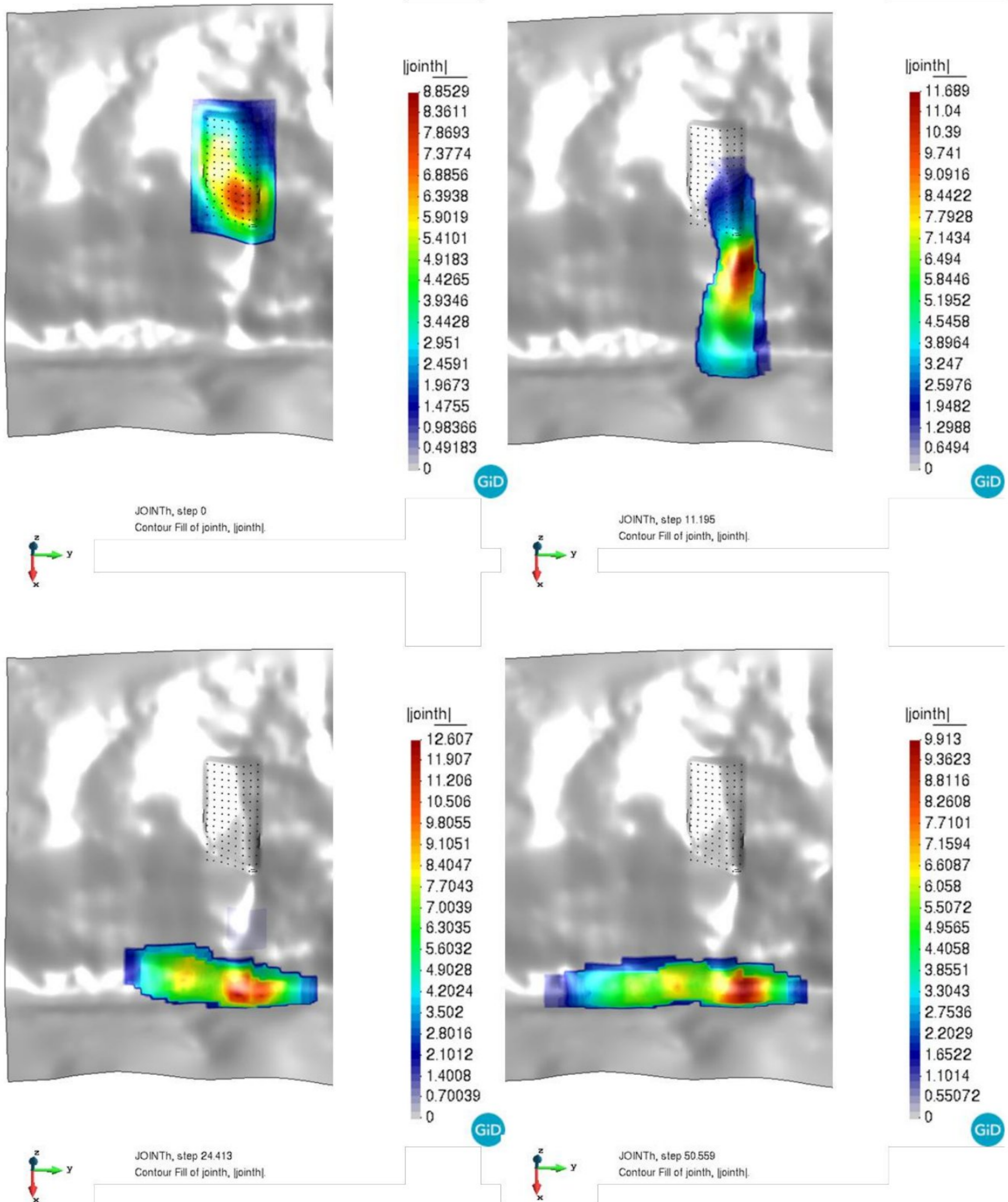
Слика 8.30 SPH 3 модел симулације кретања материјала и коначних дубина депоновања тежишта Лева река
