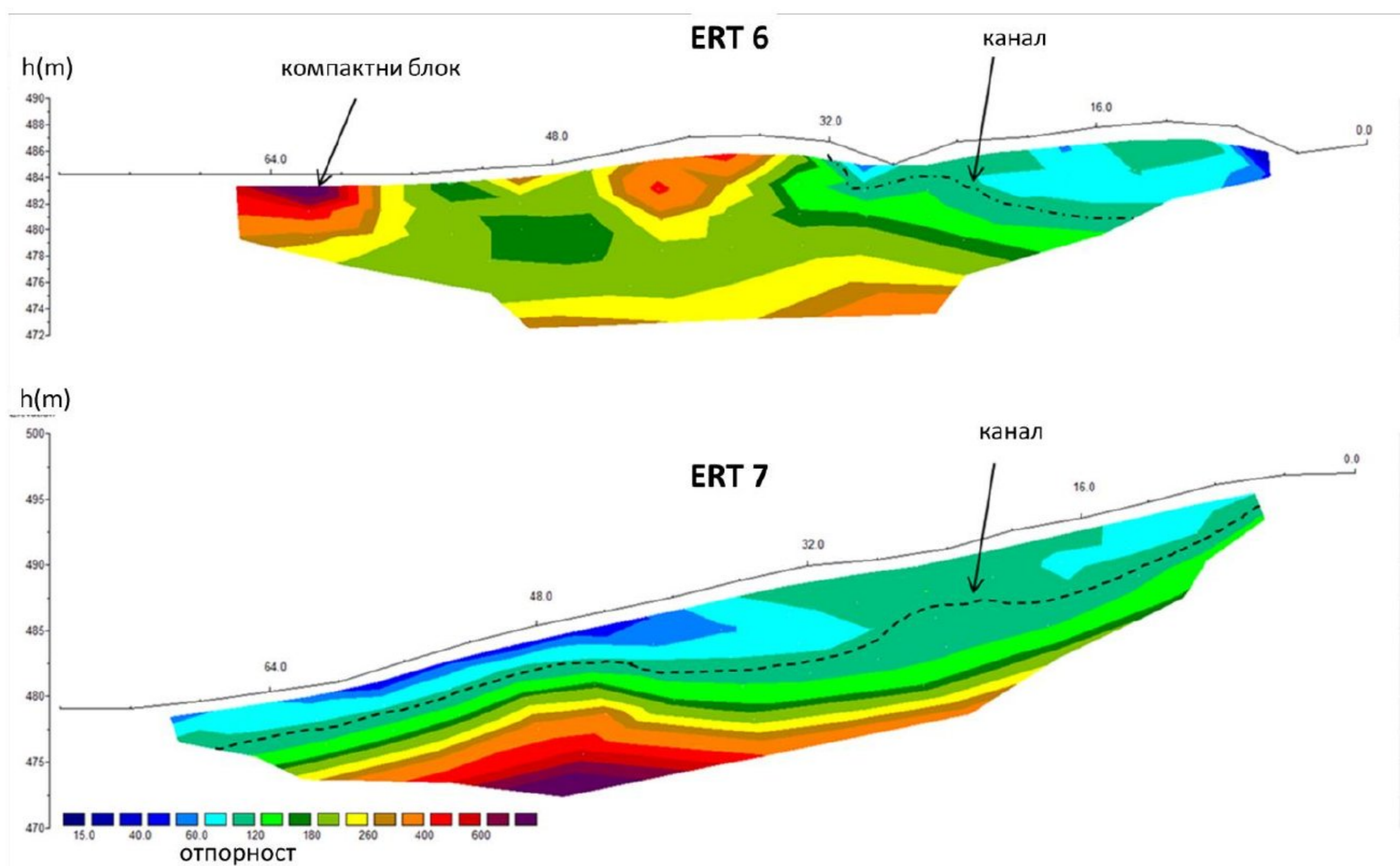
Слика 6.13 Резултати ERT 6 и ERT 7 профила
