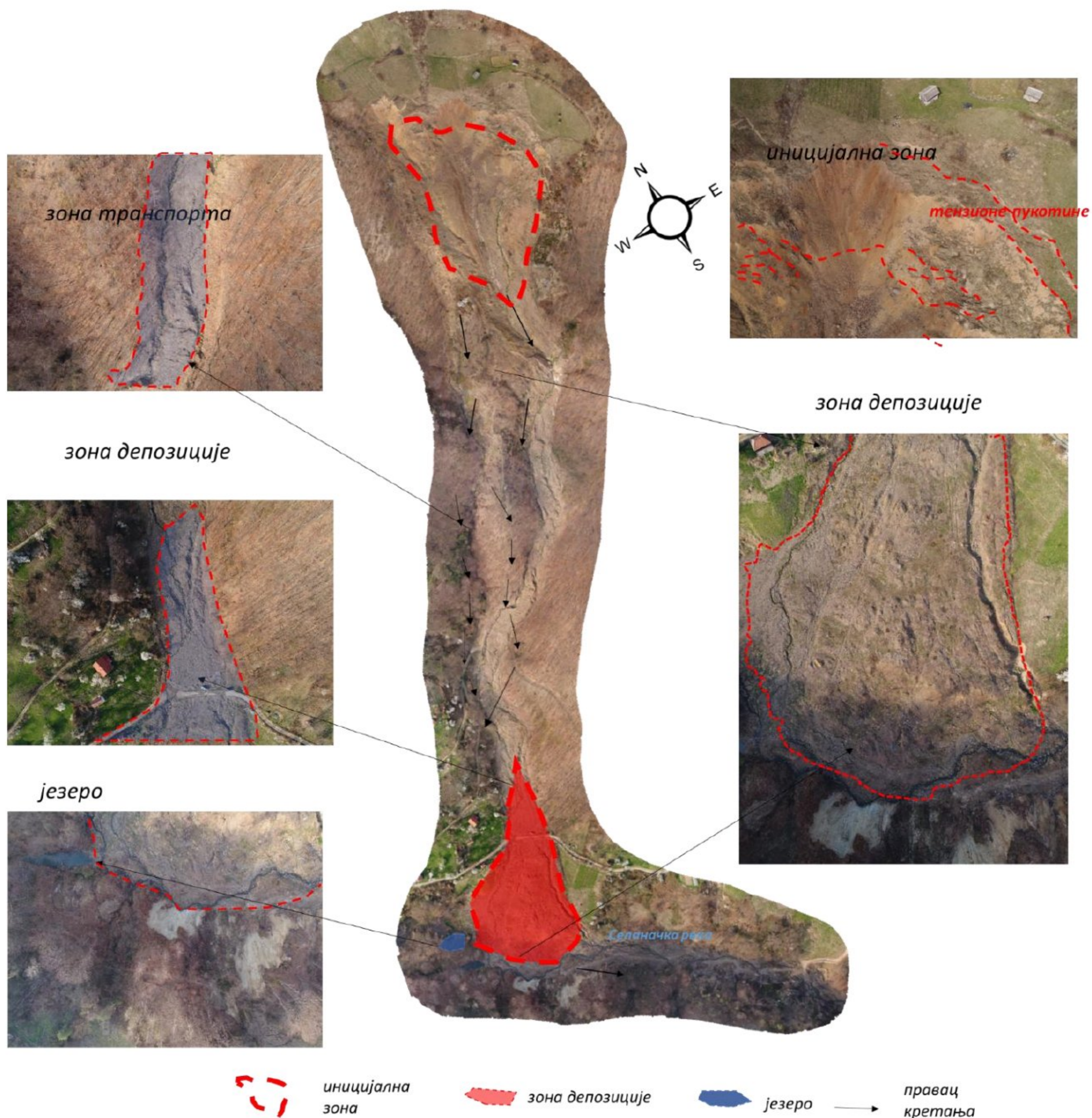
Слика 6.1 Ортофото снимак тецишта Селанац добијен UAV фотограметријским снимањем са карактеризацијом основних геометријских елемената
