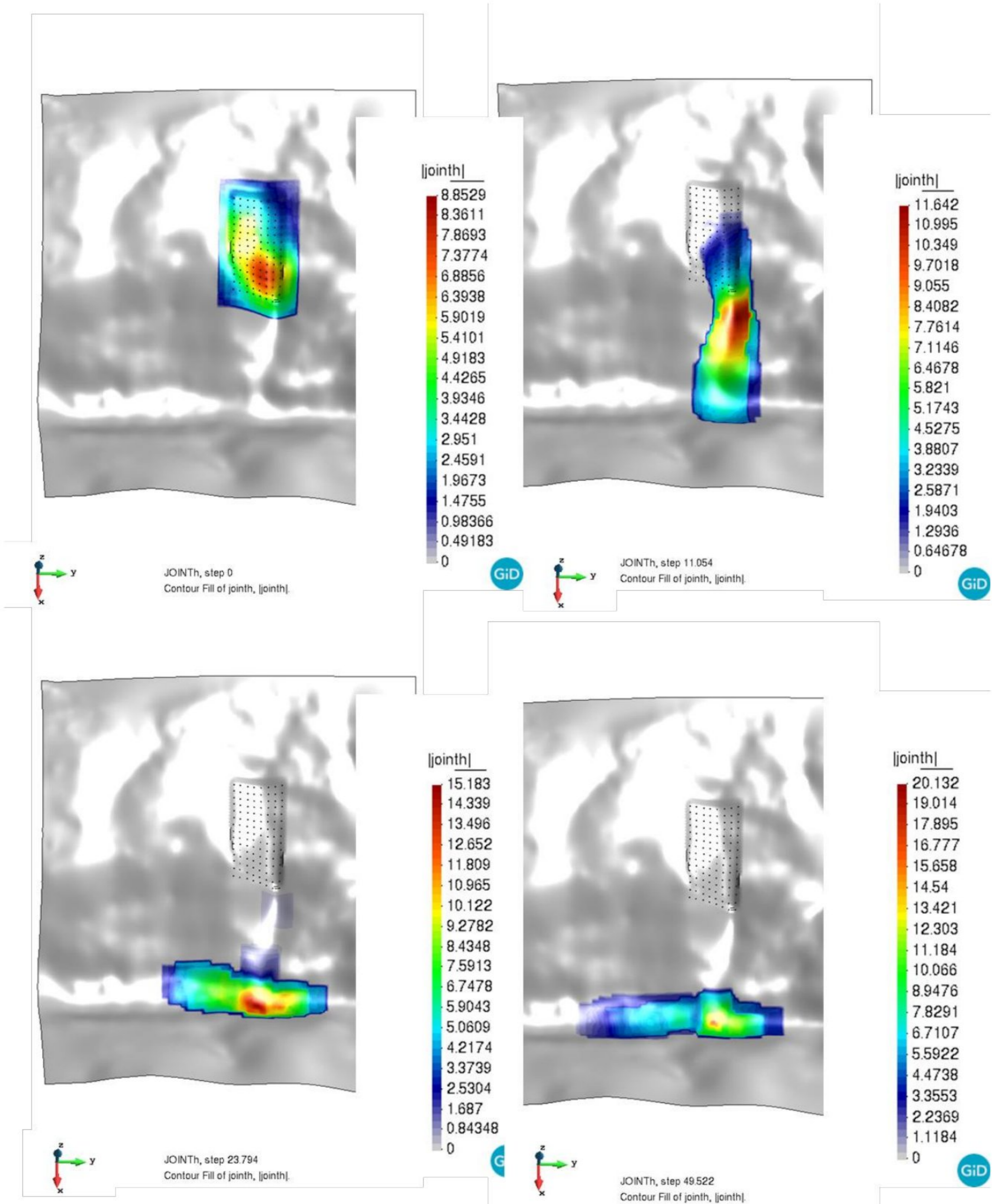
Слика 8.24 SPH 1 модел симулације кретања материјала и коначних дубина депоновања тецишта Лева река
