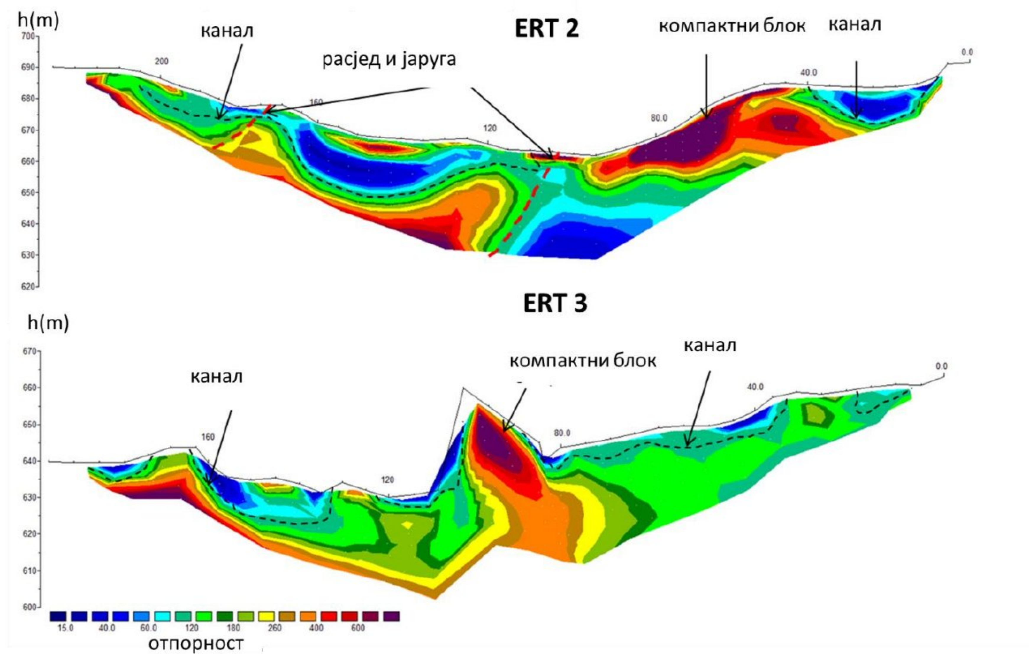
Слика 6.11 Резултати ERT_2 и ERT_3 профила
