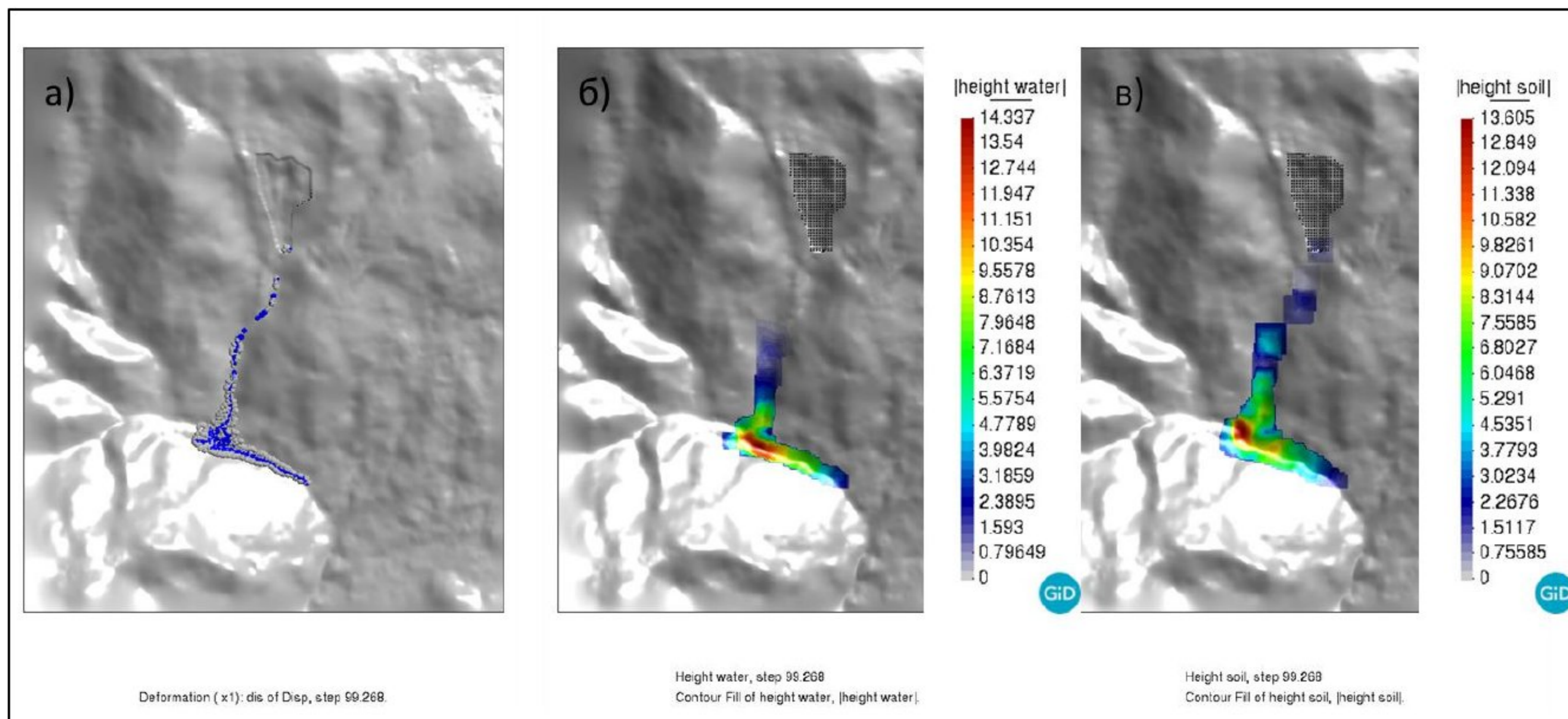
Слика 8.16 Модел SPH3 а) према параметру помјерања фаза б) висина флуидне фазе в) висина чврсте фазе
