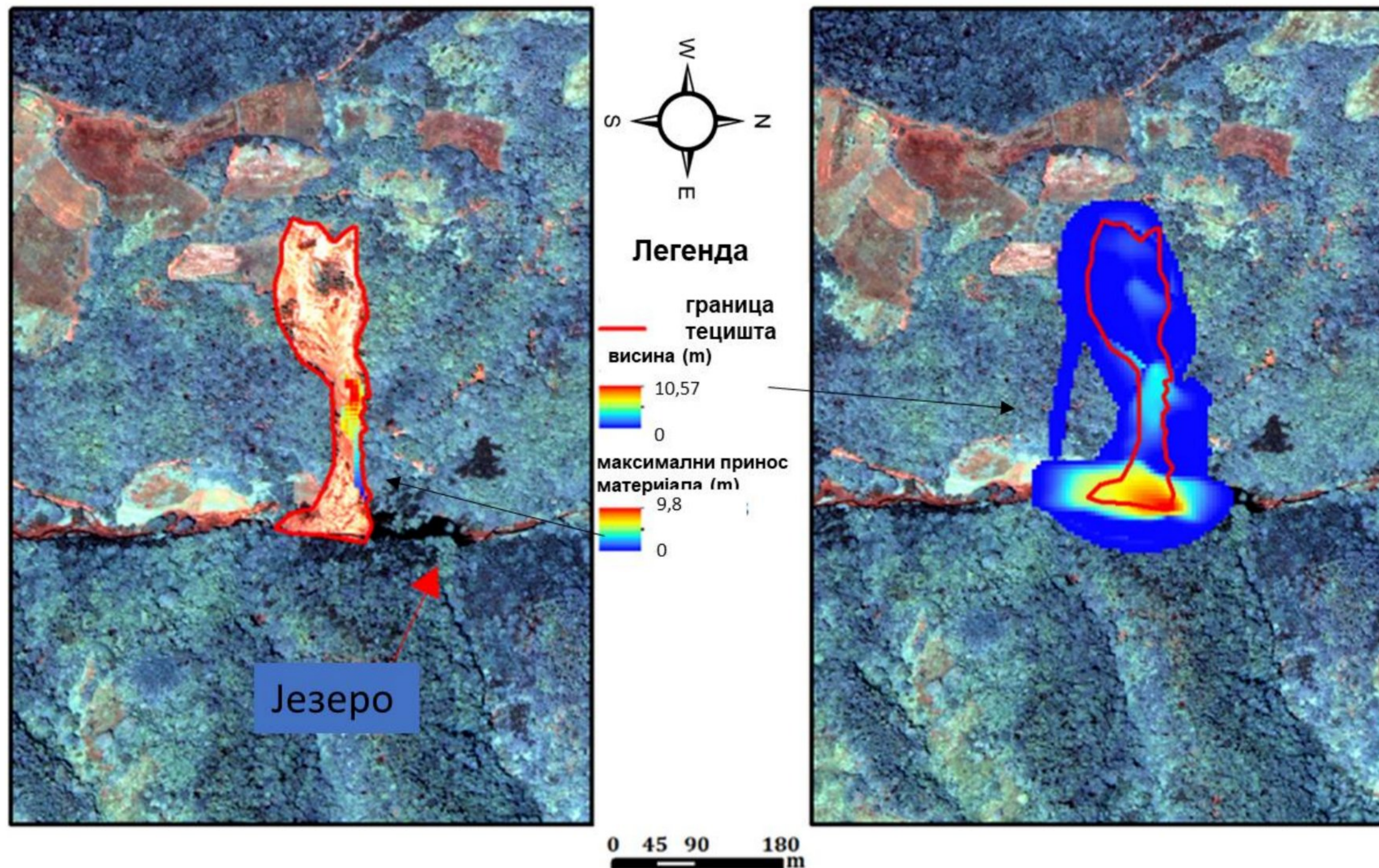
Слика 8.21 Модел финалних дубина тецишта Лева река на прецизнијем моделу терена са прорачуном приноса материјала (Крушић et. al., 2018)
