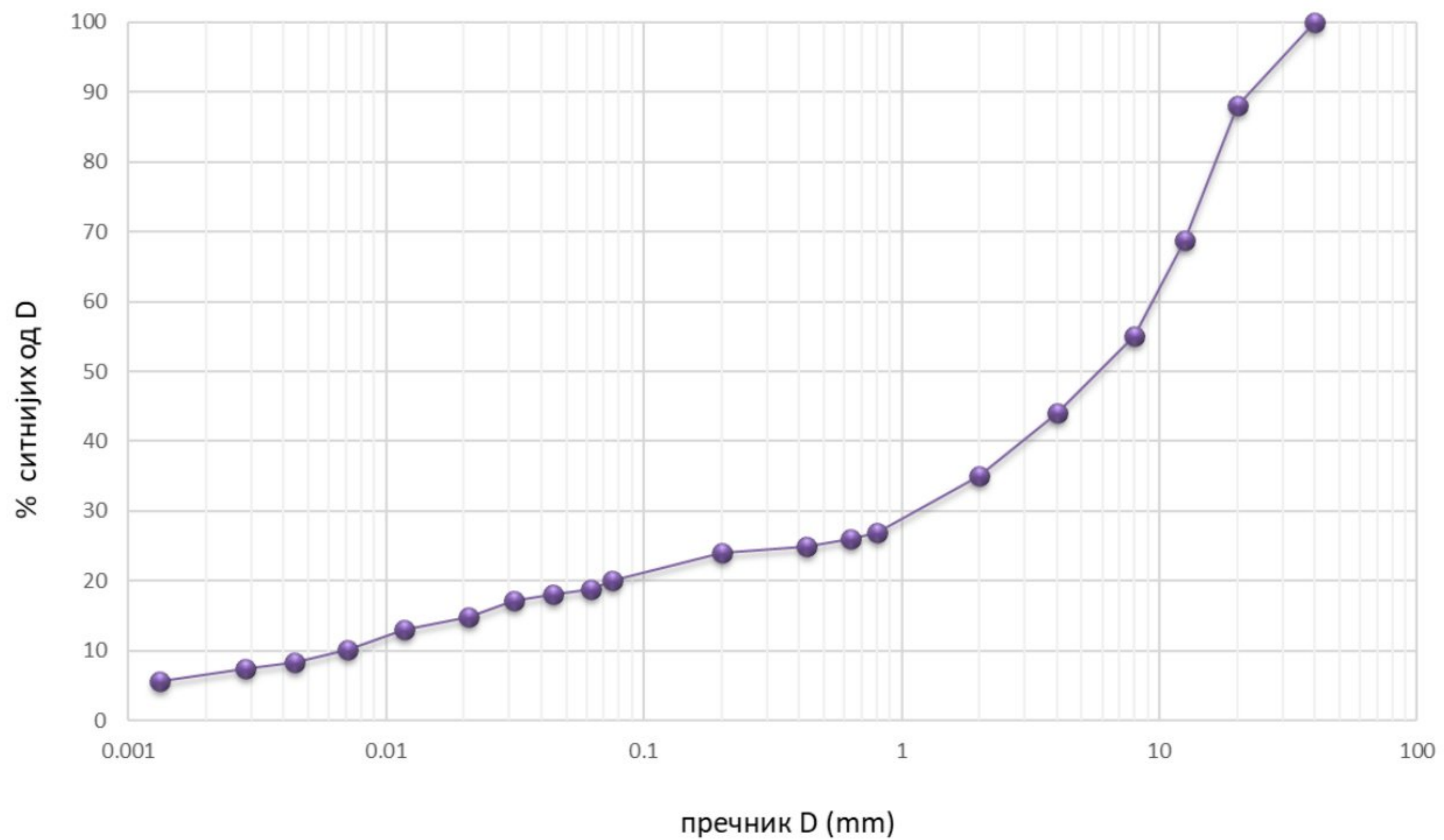
Слика 7.5 Резултати опита добијања мијешане криве сијањем и хидрометрисањем на узорку LM-1
