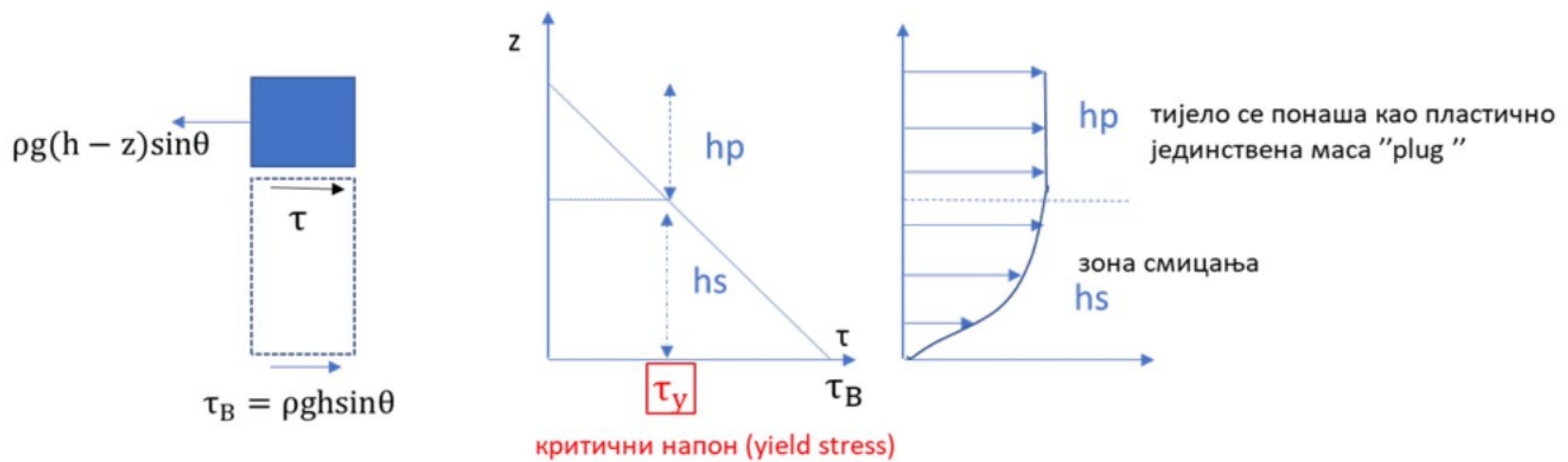
Слика 2.10 Бингамов модел понашања приликом течења
