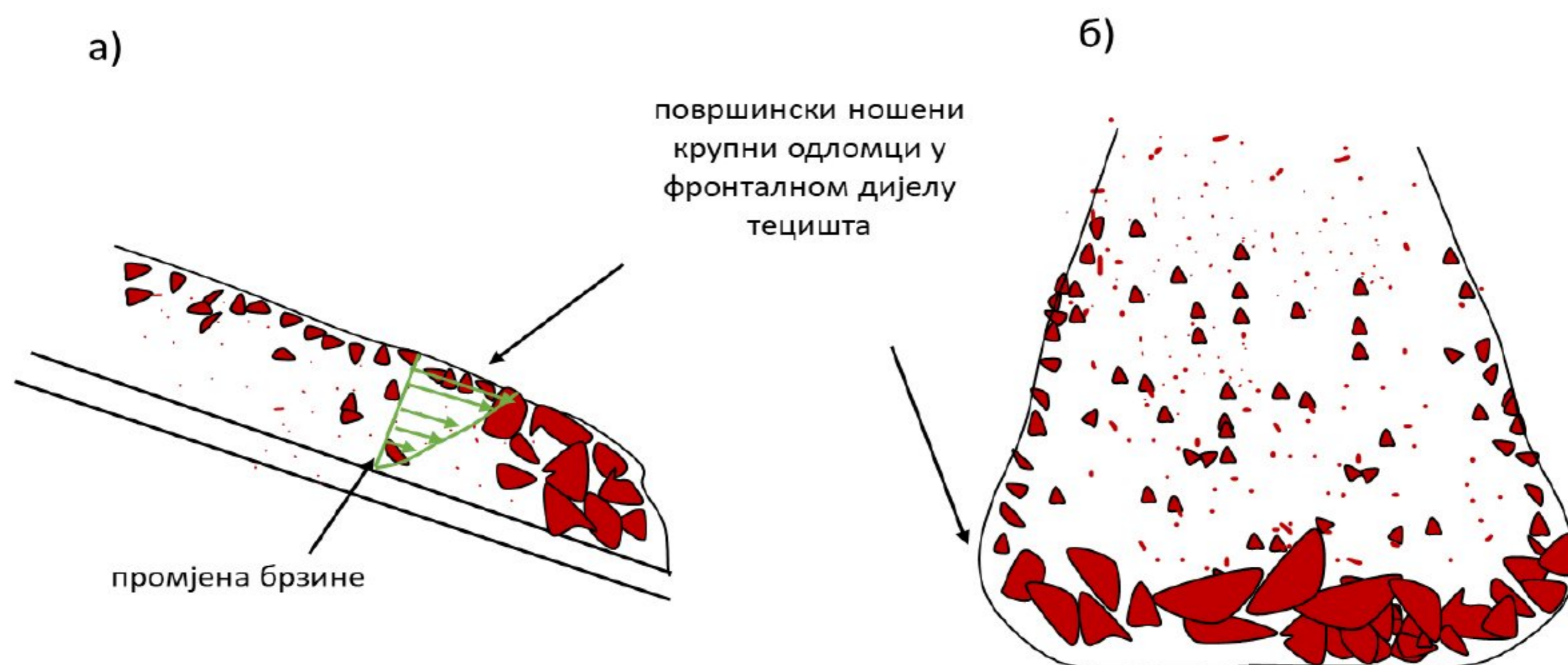
Слика 2.5 Приказ тецишта а) у пресјеку и б) у плану са карактеристичним таложењем материјала
