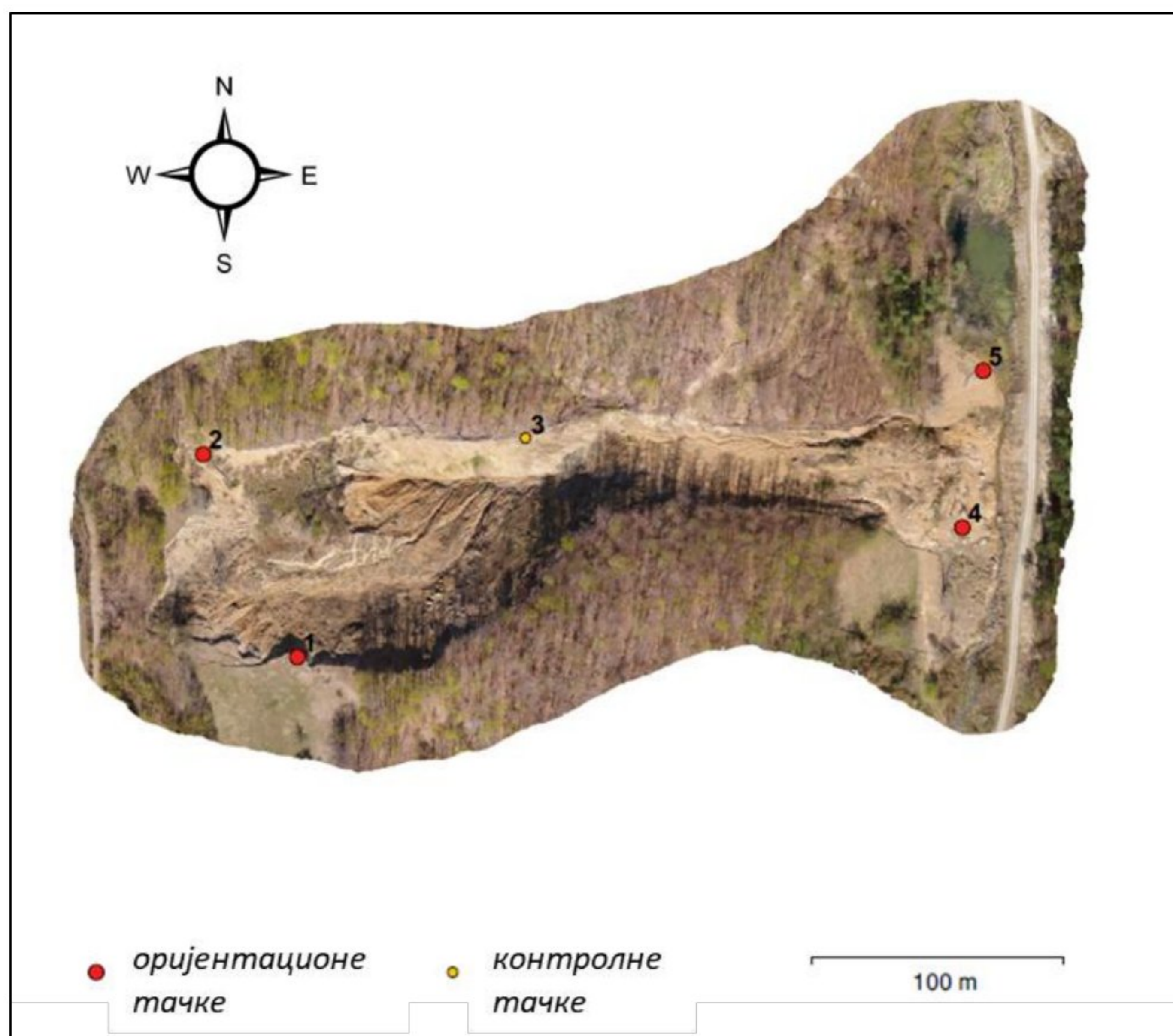
Слика 6.17 Положај оријентационих и контролних тачака
