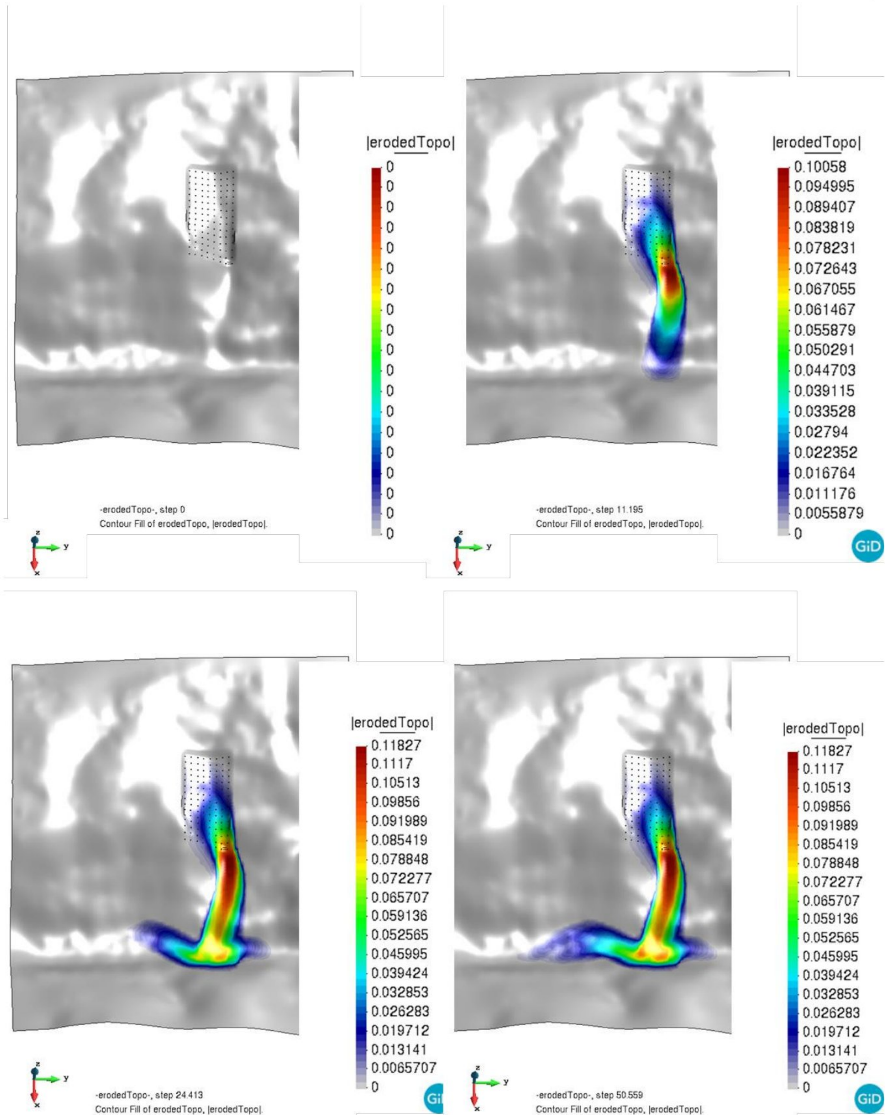
Слика 8.31 SPH 3 модел прорачуна степена приноса материјала ег у зони транспорта тежишта Лева река
