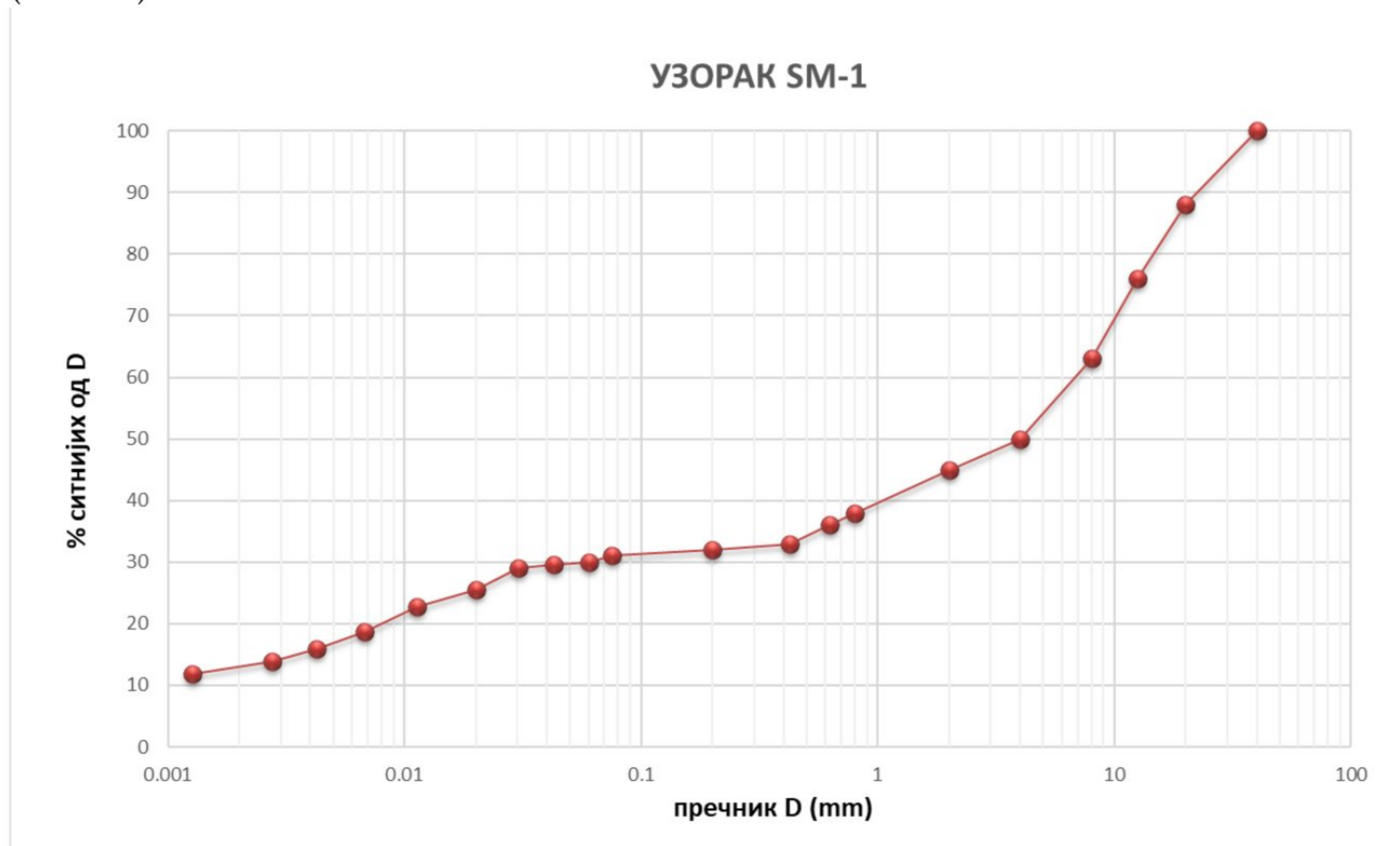
Слика 7.2 Резултати опита добијања мијешане криве ситањем и хидрометрисањем на узорку SM-1
