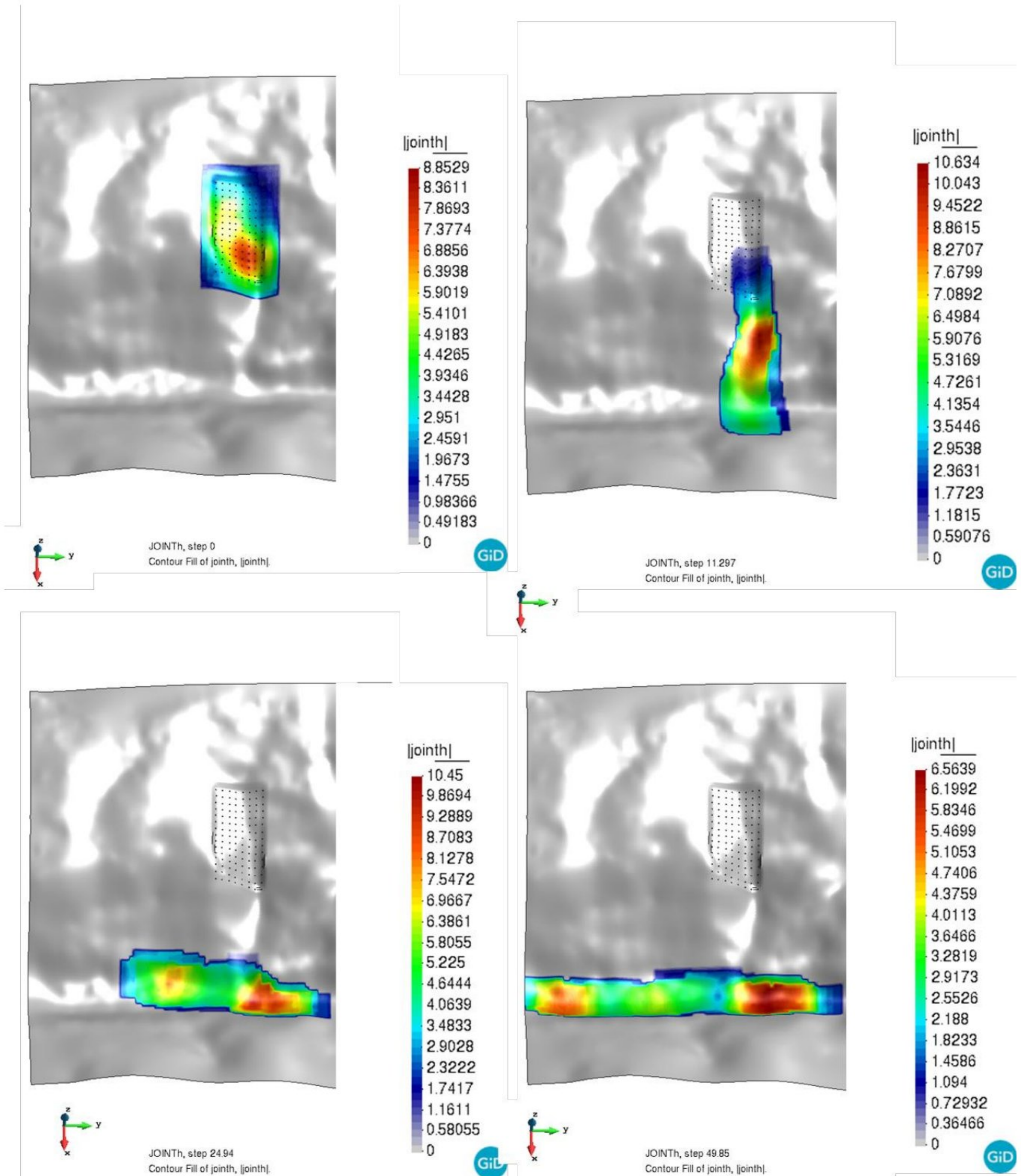
Слика 8.27 SPH 2 модел симулације кретања материјала и коначних дубина депоновања тежишта Лева река
