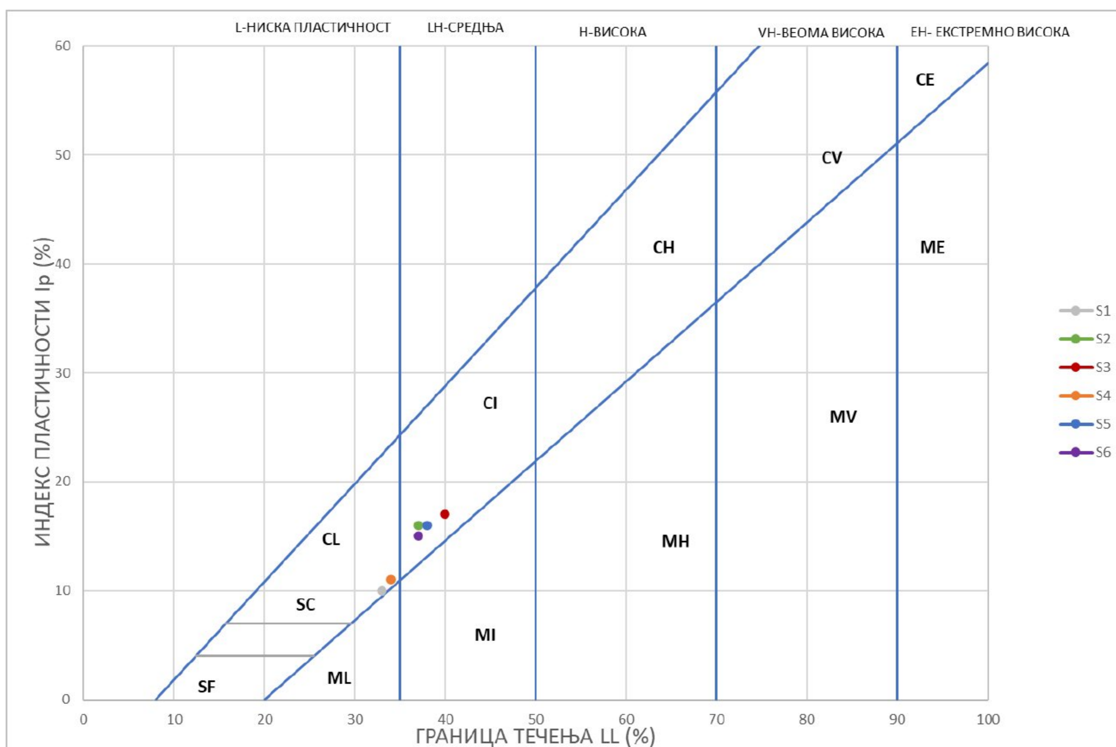
Слика 7.4 USCS дијаграм на основу параметара конзистенције
