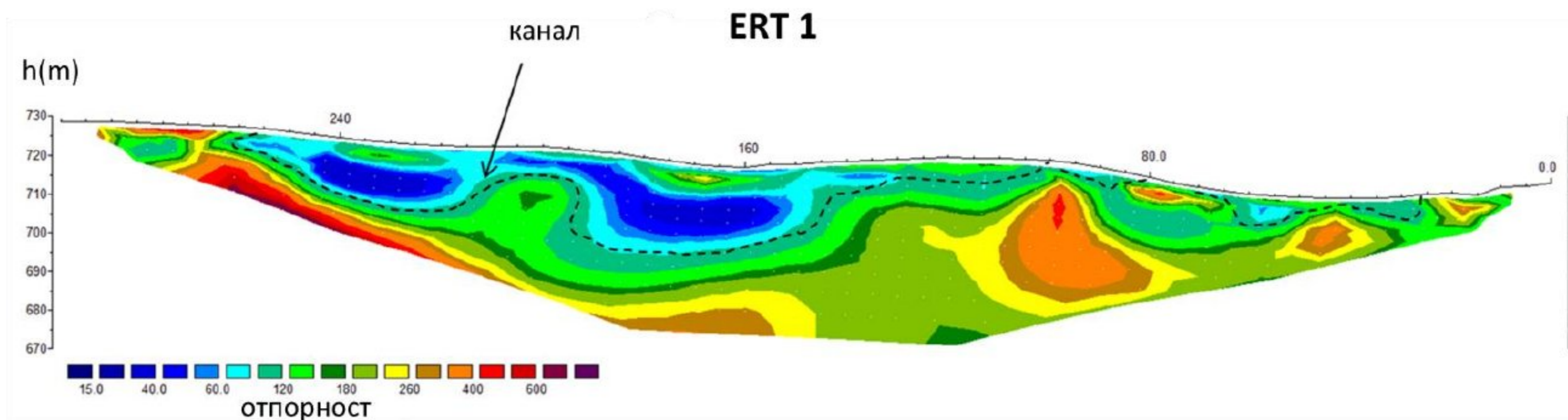
Слика 6.10 Резултати ERT_1 профила
