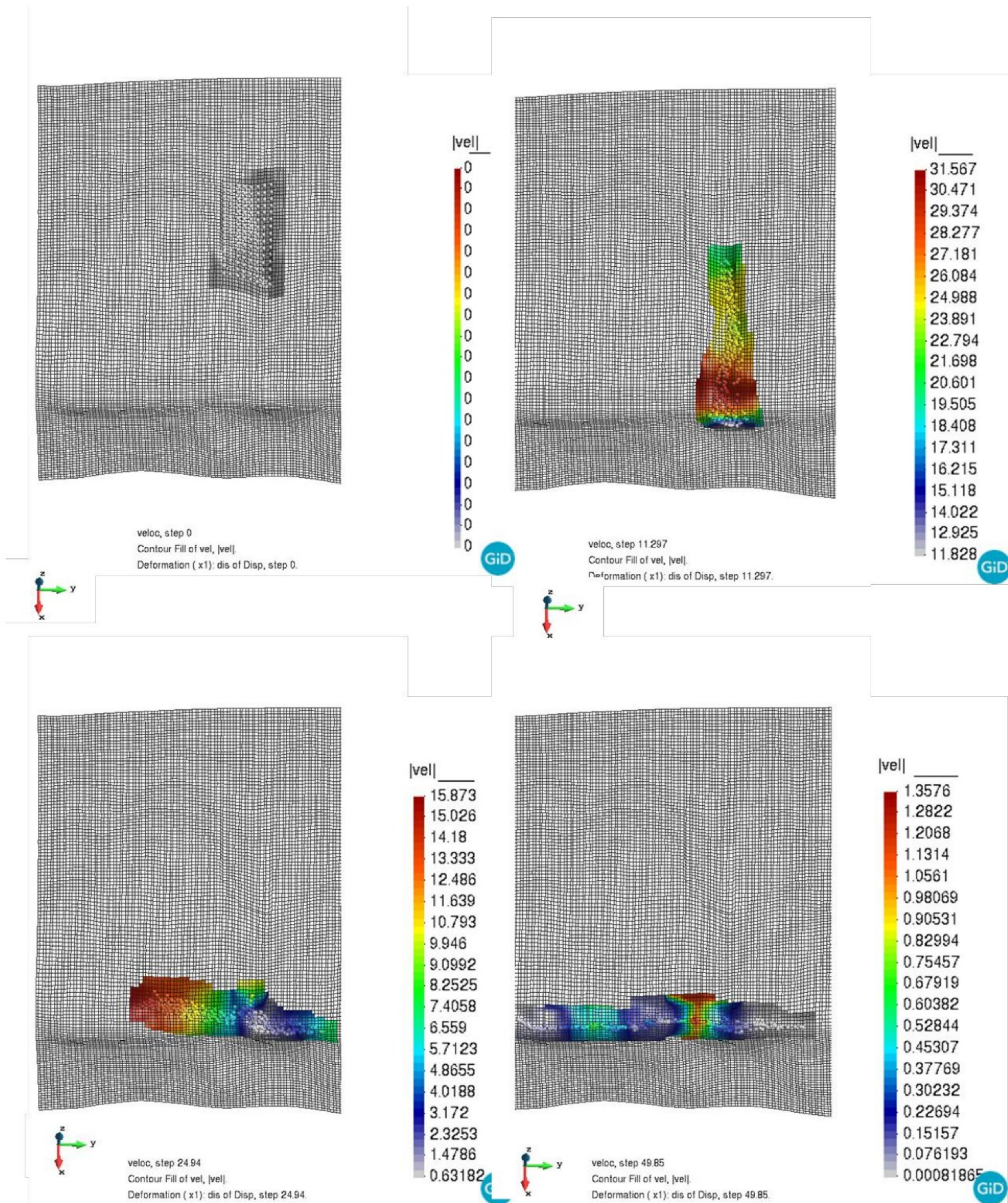
Слика 8.29 SPH 2 модел прорачуна достигнутих максималних брзина течења тецишта Лева река
