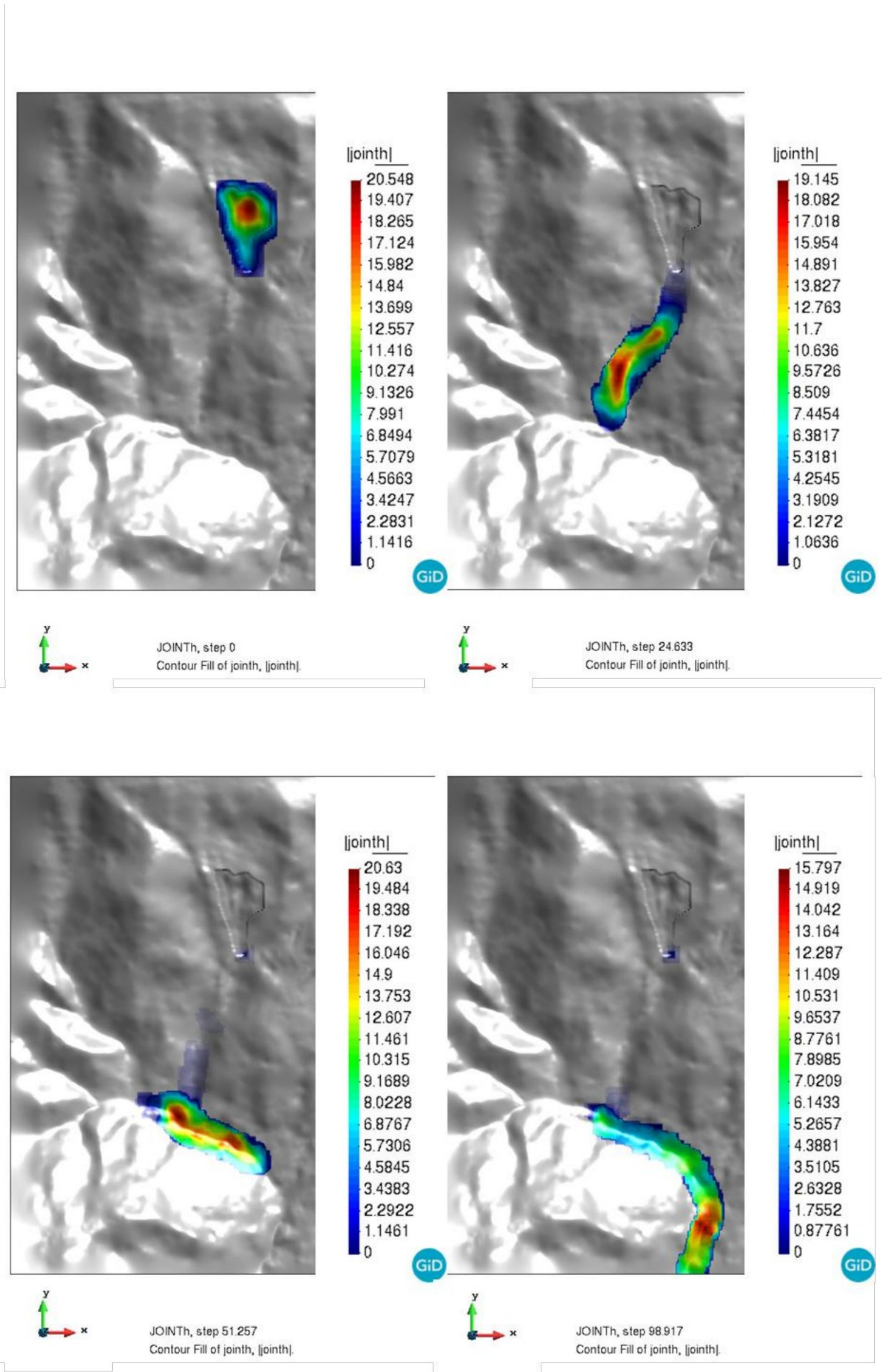
Слика 8.7 SPH1 модел симулације кретања материјала и коначних дубина депоновања
