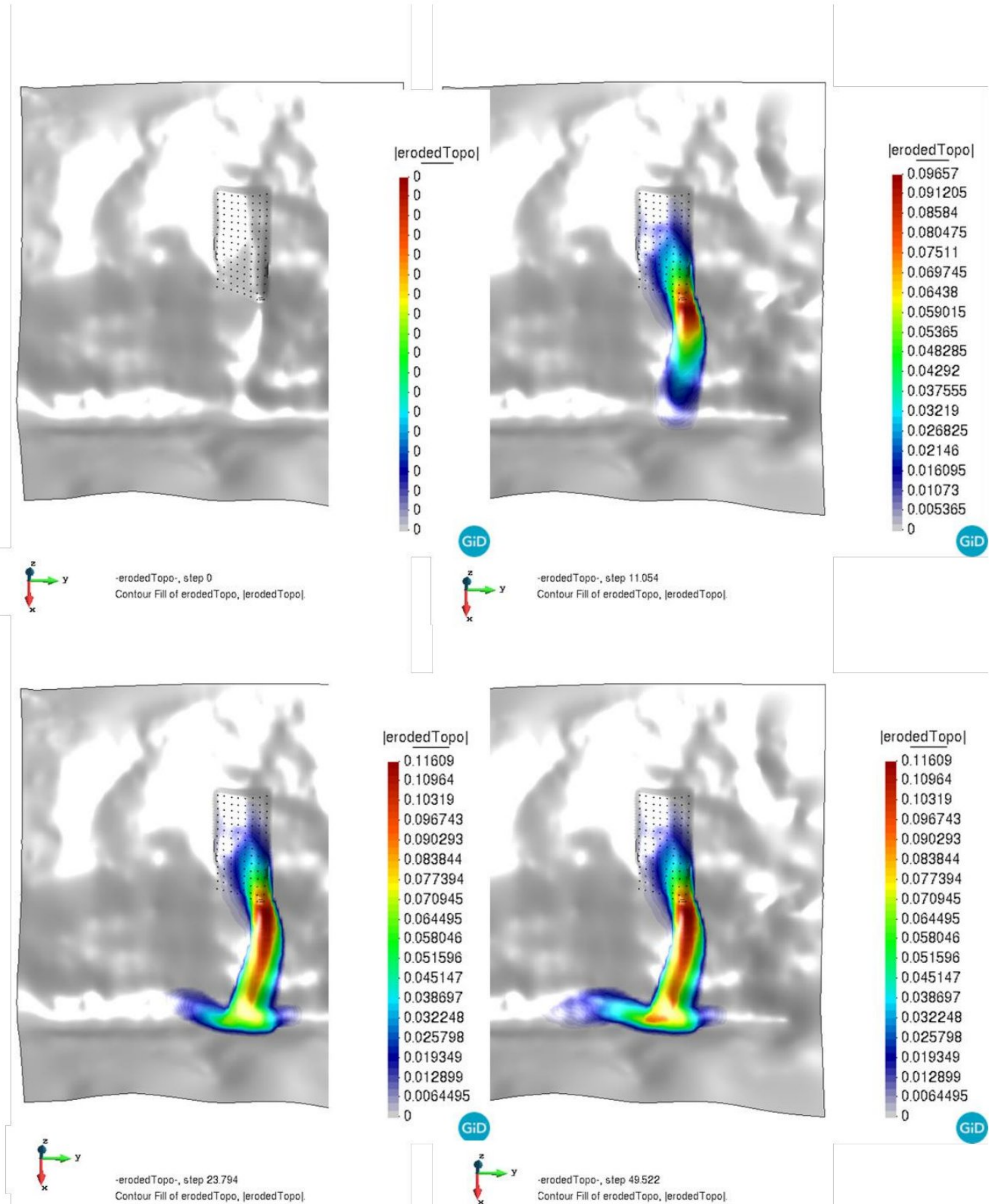
Слика 8.25 SPH 1 модел прорачуна степена приноса материјала ег у зони транспорта тежишта Лева река
