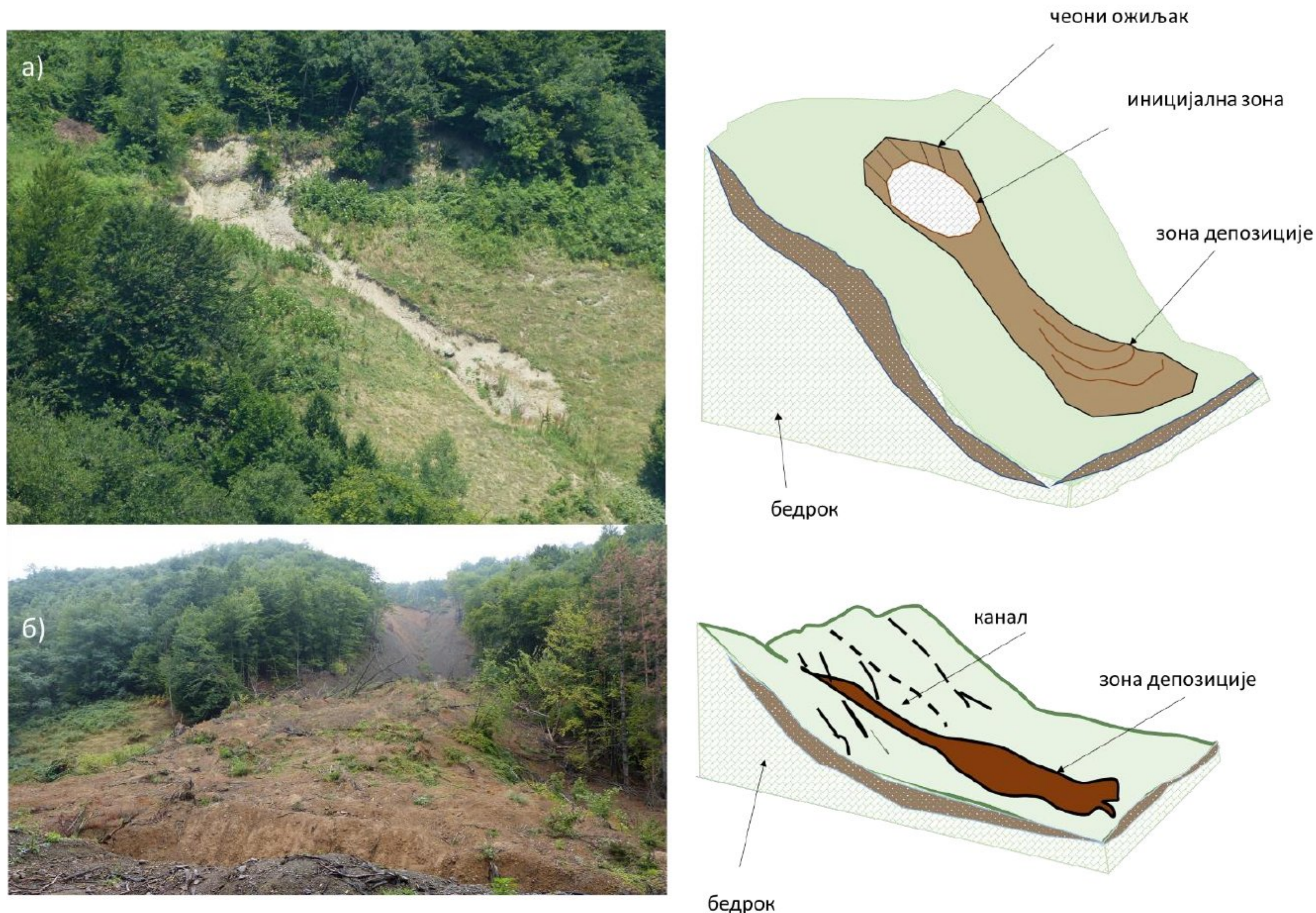
Слика 2.4 Примјери тецишта са скицама основних геометријских елемената: а) плитко тециште регистровано у Бајиној Башти на стрмој падини б) тециште Лева река код Краљева формирано у јарузи
