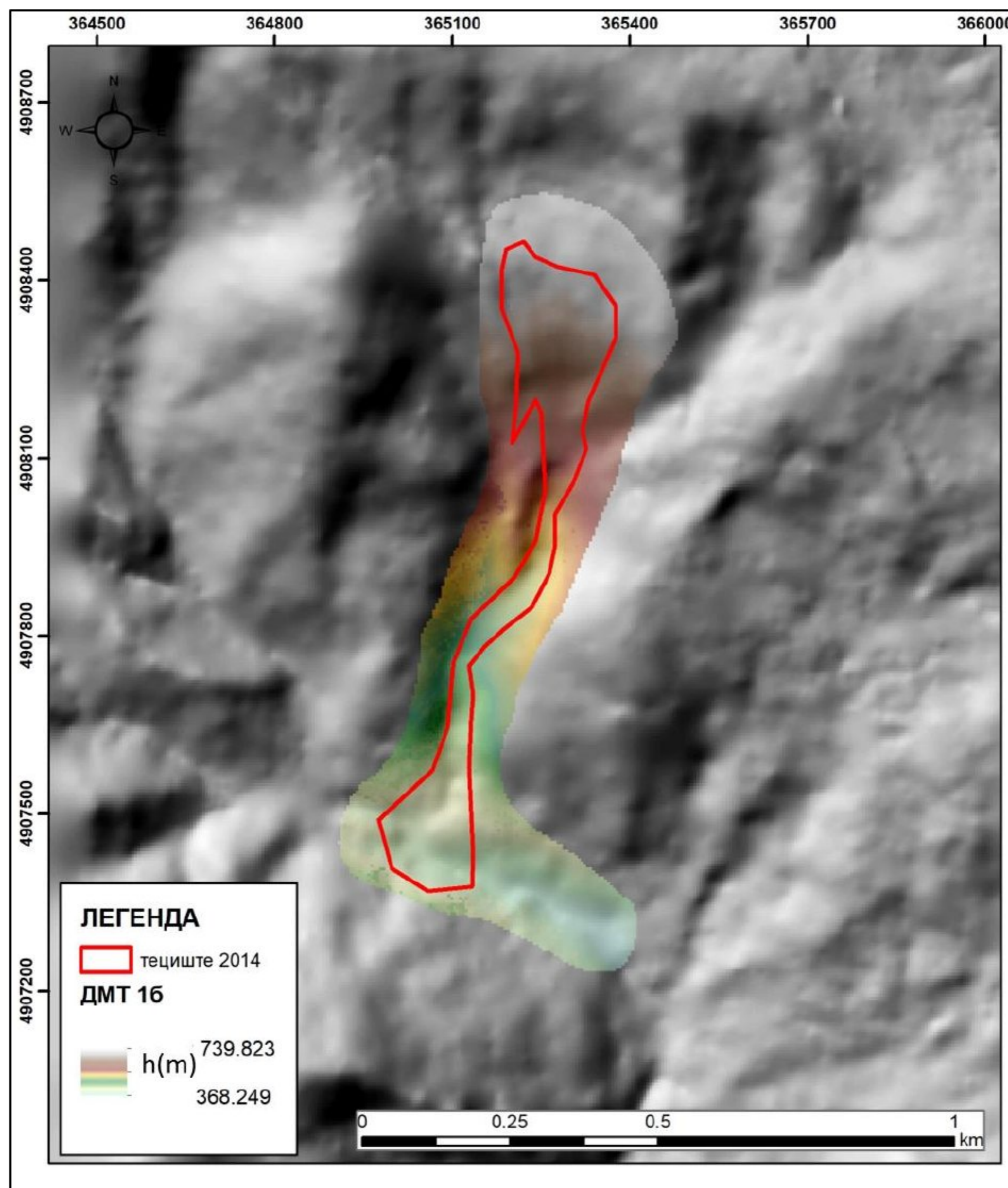
Слика 6.8 Дигитални модел терена 5x5m (изведен из модела 10x10 ст ) са уцртаним положајем активираниог тецишта Селанац
