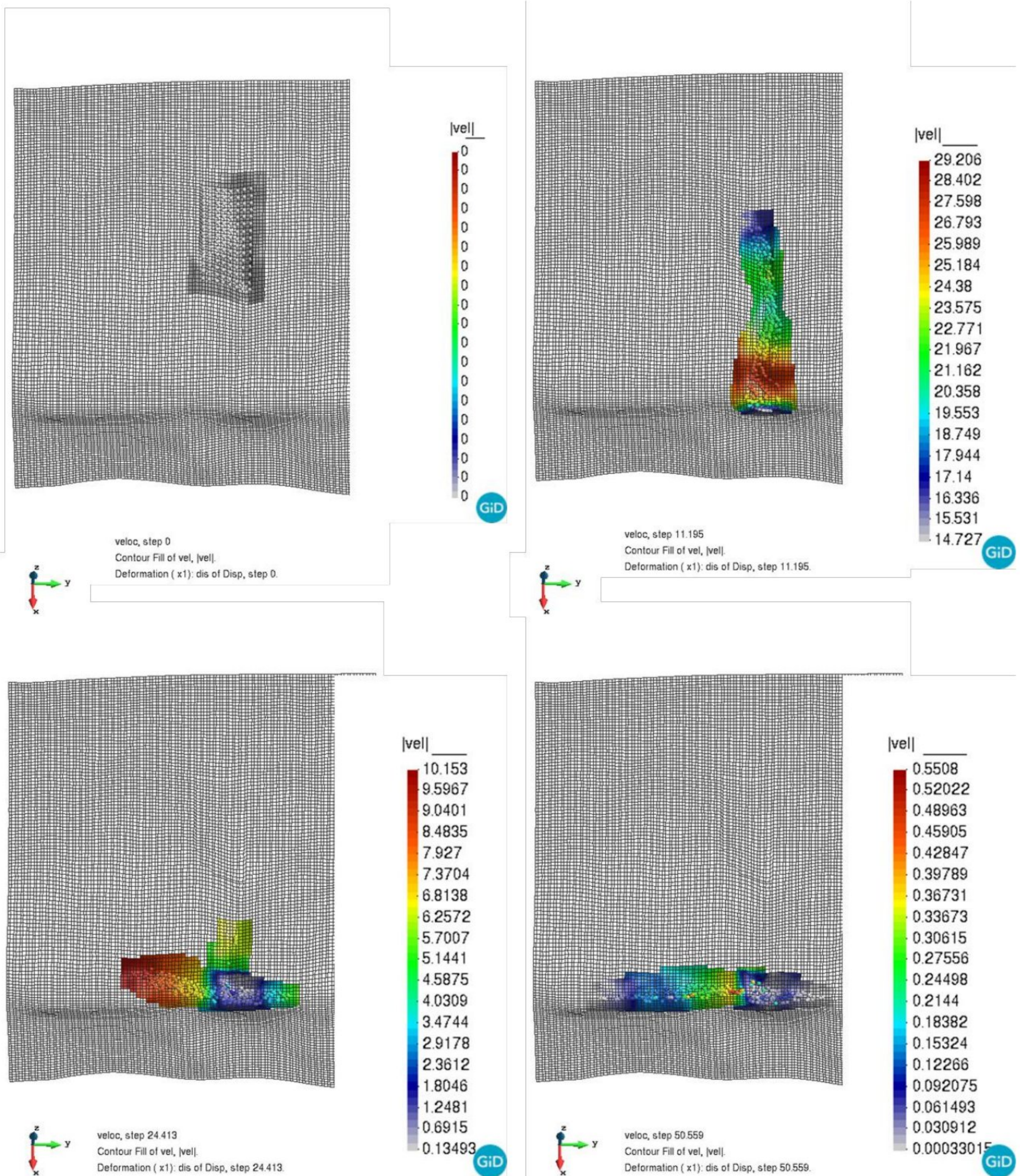
Слика 8.32 SPH 3 модел прорачуна достигнутих максималних брзина течења тежишта Лева река
