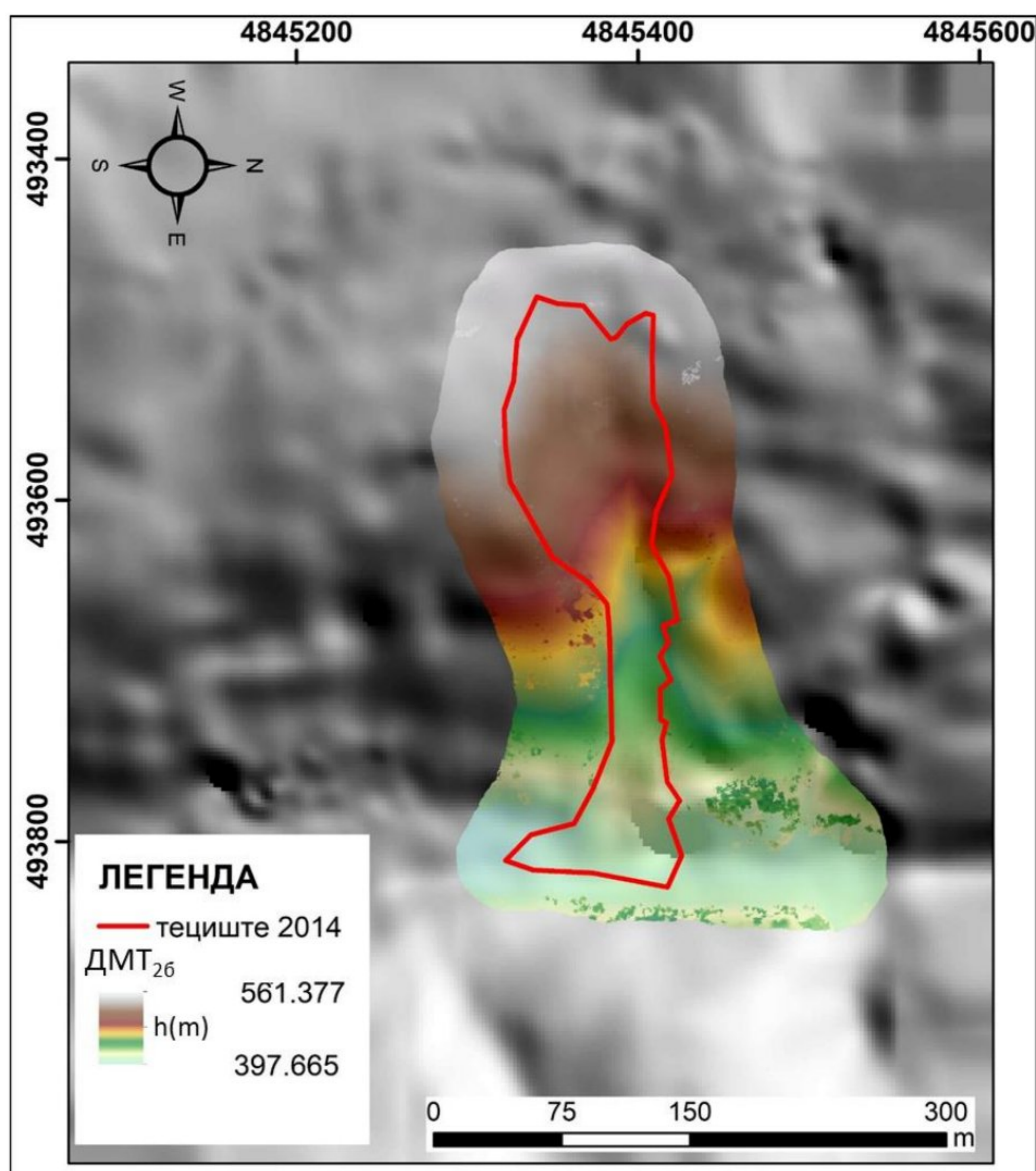
Слика 6.18 Дигитални модел терена ДМТ 26 10x10 ст са уцртаним положајем активираниог тецишта Лева река
