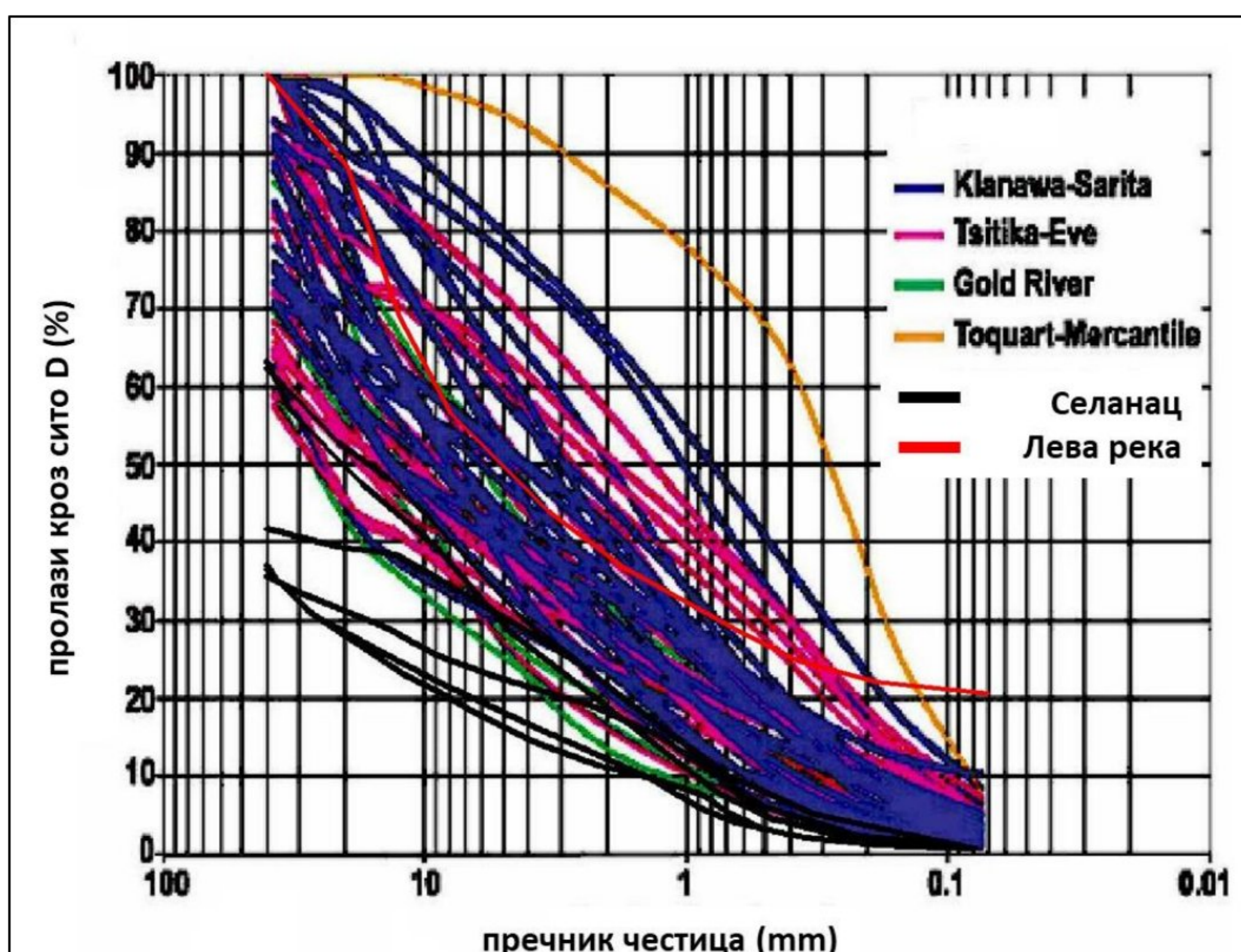
Слика 7.8 Поређење резултата гранулометријског састава са резултатима Brideau et.al, 2019
