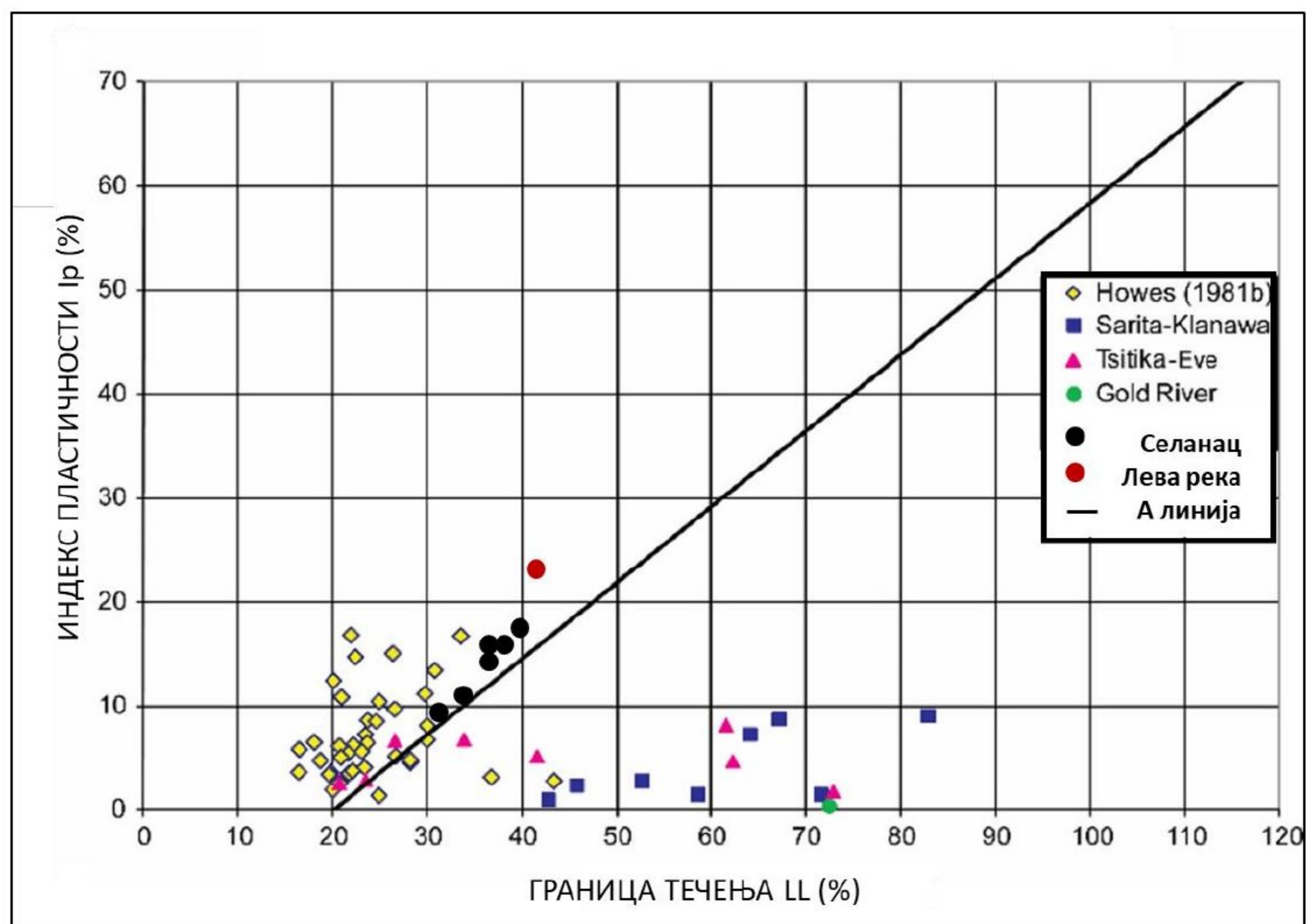
Слика 7.9 Поређење резултата опита конуса пенетрације са резултатима Brideau et.al, 2019
