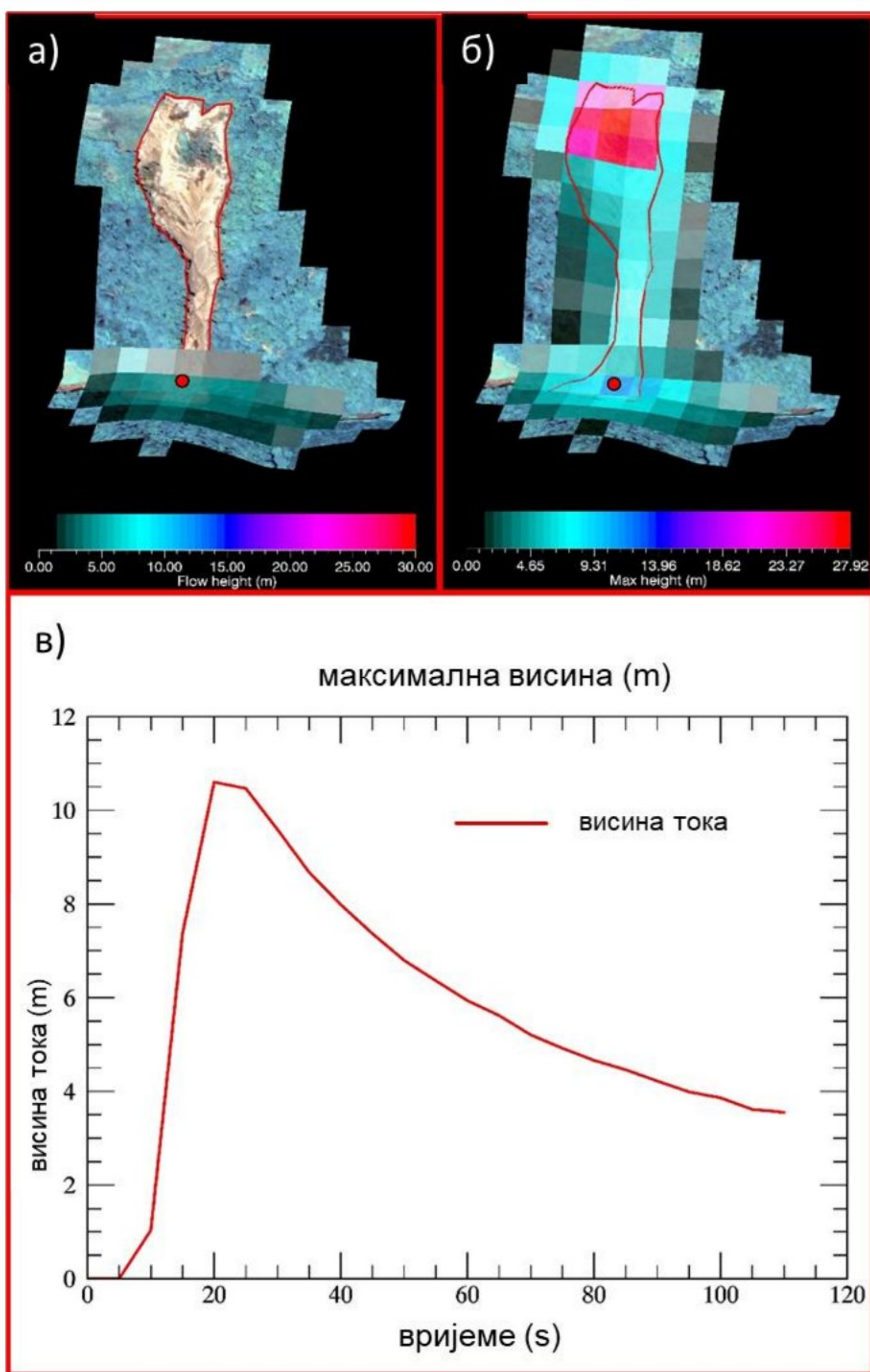
Слика 8.18 Прелиминарни модел са приказом а) финалних дубина б) максималних висина тока в) промјене висине тока у тачки (Крушић, et al. (2017))
