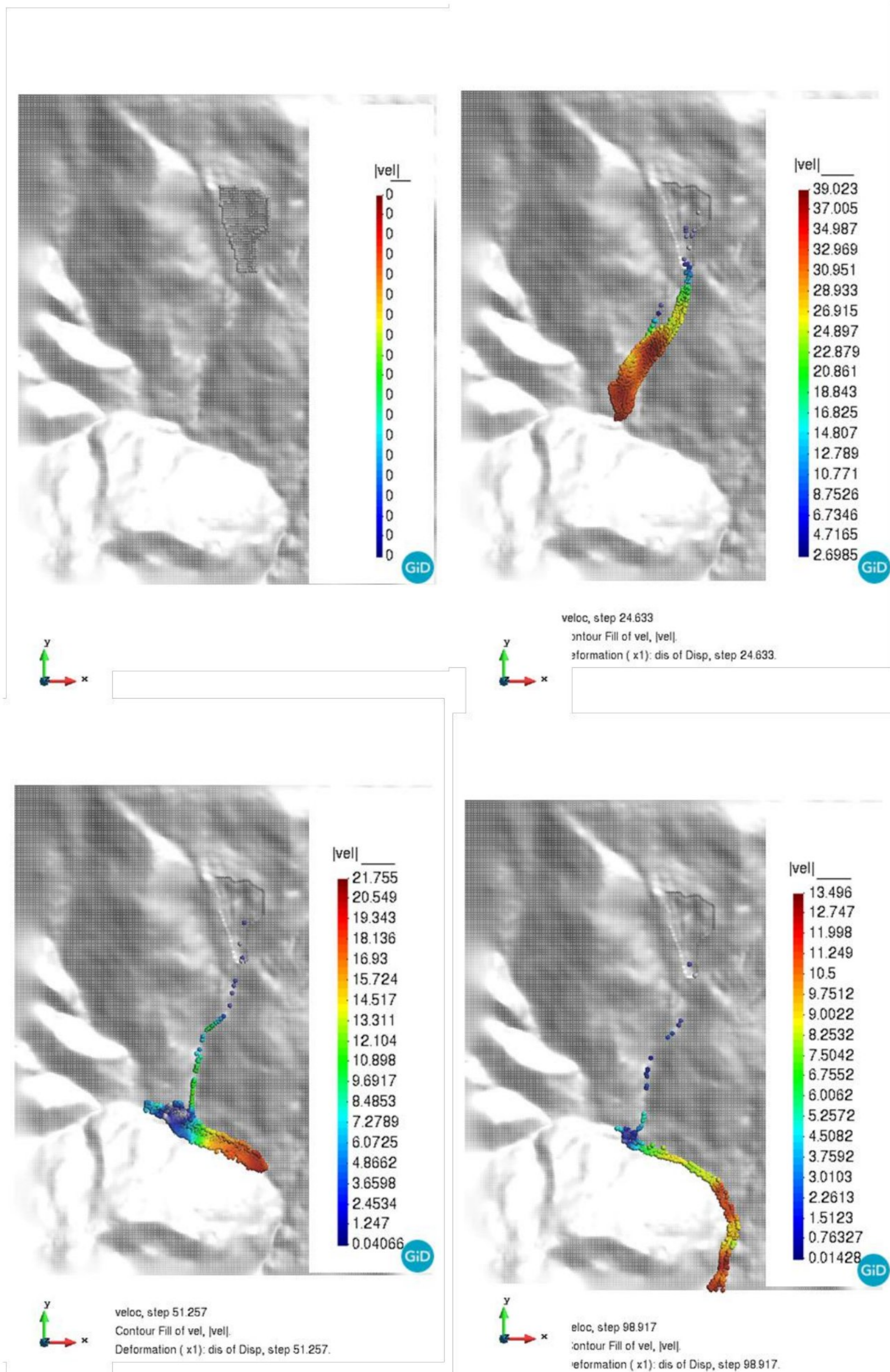
Слика 8.9 SPH1 модел прорачуна достигнутих максималних брзина течења
