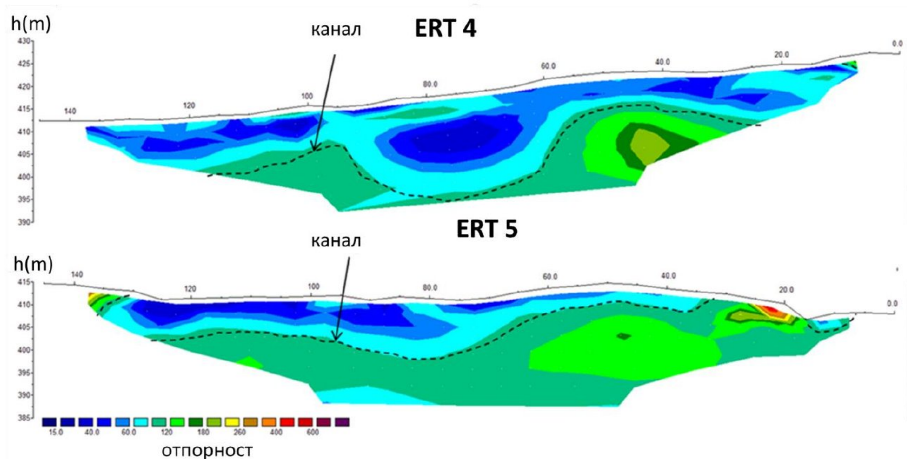
Слика 6.12 Резултати ERT 4 и ERT 5 профила
