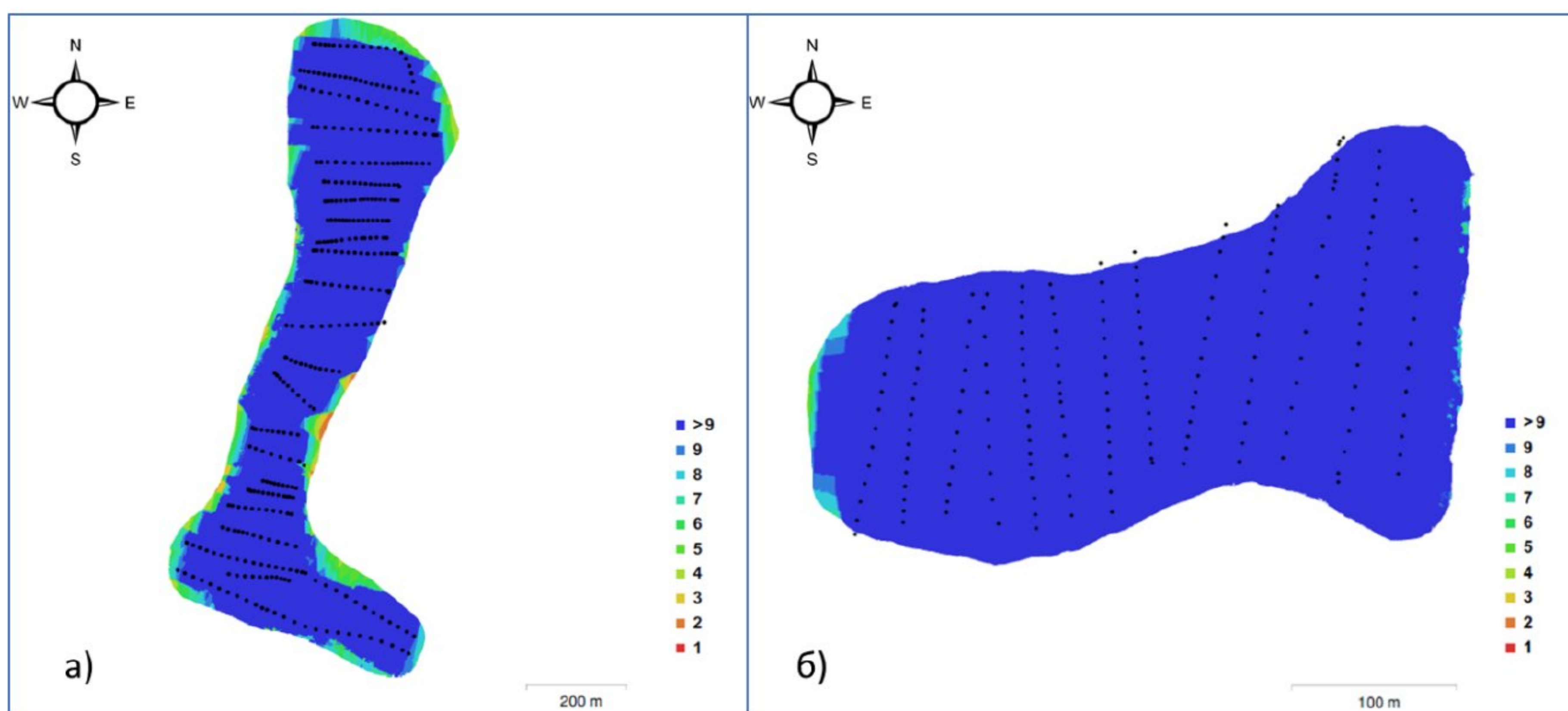
Слика 4.2 Позиција камере и преклапања снимака а) тециште Селанац б) тециште Лева река
