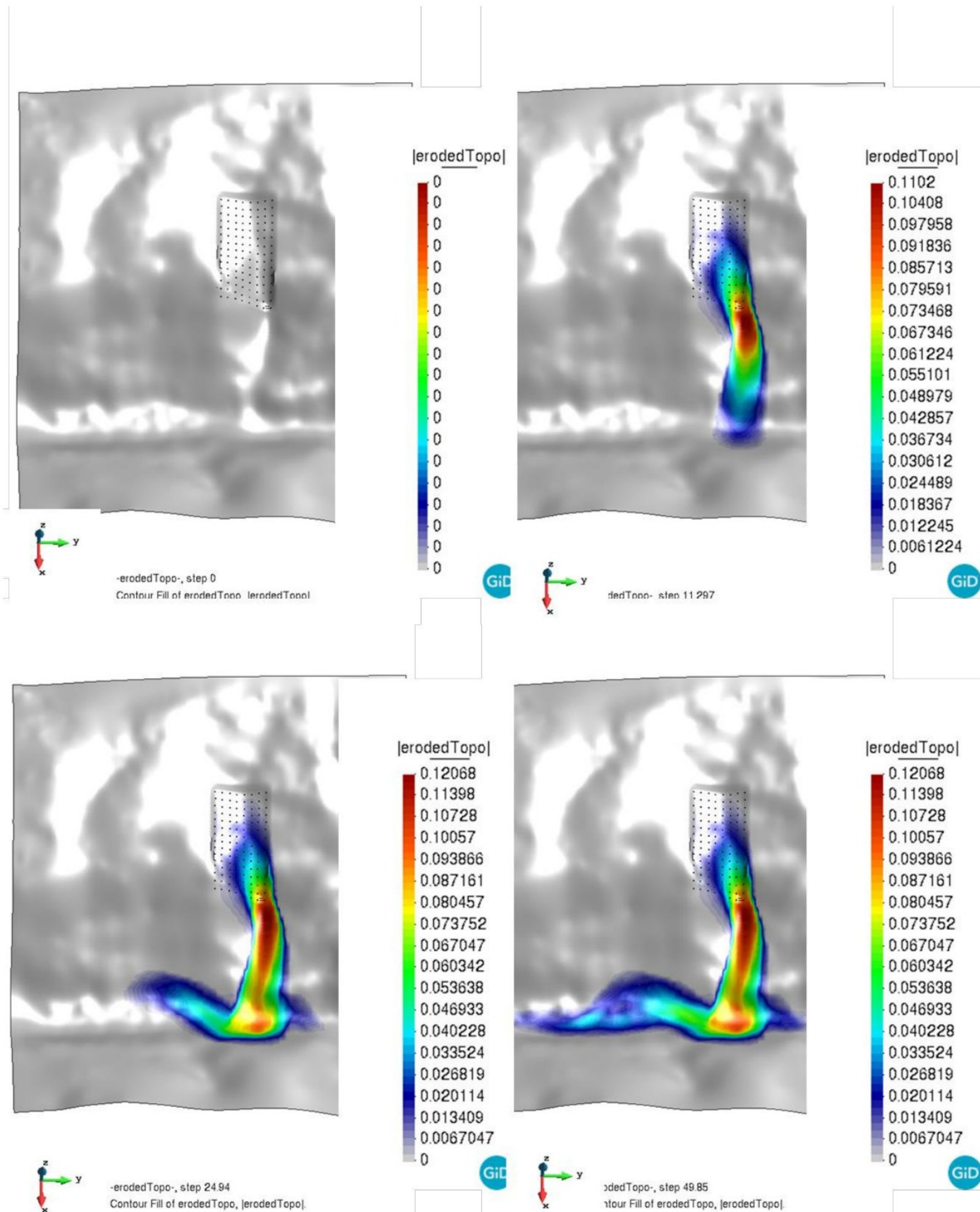
Слика 8.28 SPH 2 модел прорачуна степена приноса материјала ер у зони транспорта тежишта Лева река
