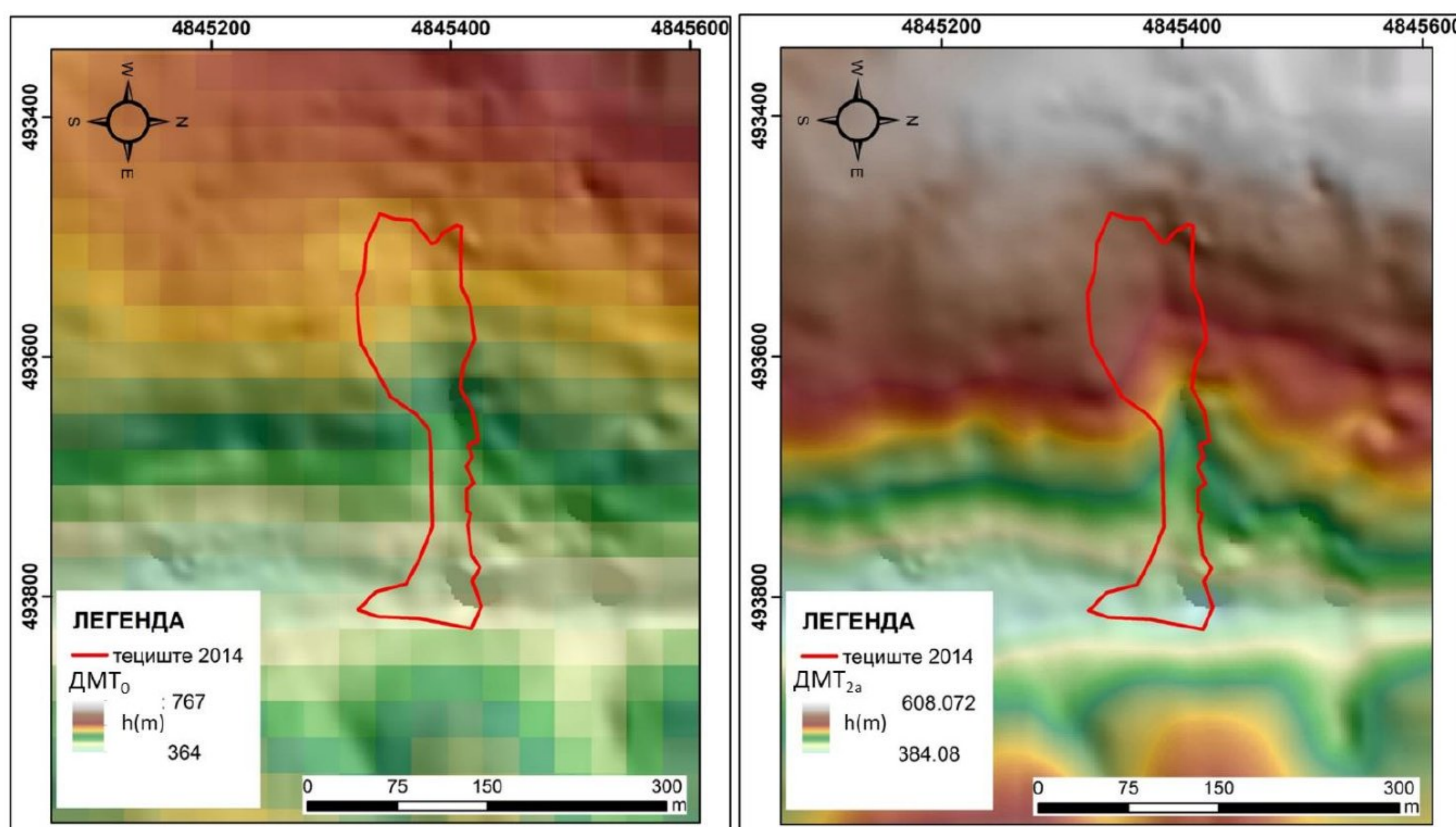
Слика 6.16 Дигитални модел терена 30x30m са уцртаним положајем накнадно активираниог тецишта
