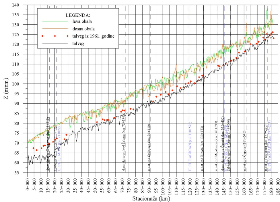
Слика 4.1.9: Упоредни уздужни профили корита Велике Мораве 1961. и 2006. године (Бабић-Младеновић и сар. 2009)
