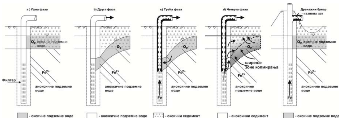
Слика 6.5: Фазе колмирања бунара услед мешања оксидичних и аноксичних подземних вода (van Beek 2012, модификовала Мајкић)
