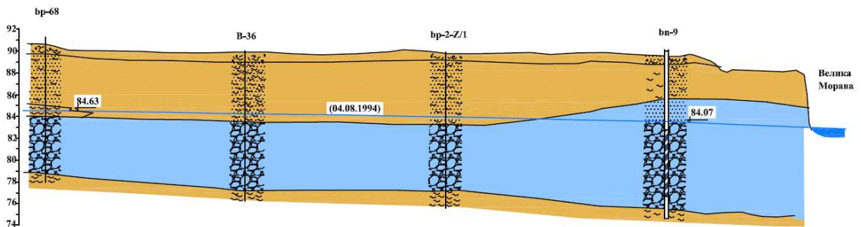
Слика 4.1.16: Хидрогеолошки профил 1-1' дуж трасе некадашњих пијезометарских бушотина вр-68 до старог бунара вп-9 (Геозавод 1994)
