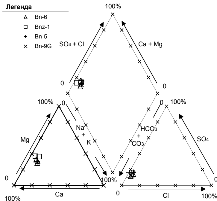
Слика 5.2: Трилинеарни дијаграм хемијског састава подземних вода изворишта Трновче
