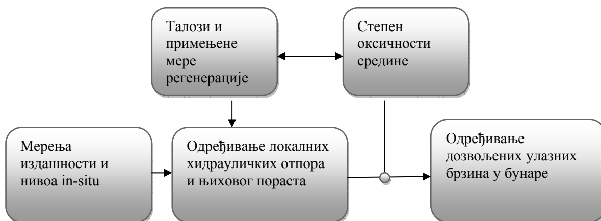
Слика 3.5: Концепт примењен при одређивању дозвољених улазних брзина у бунаре
