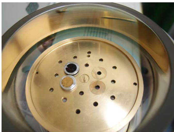
Слика 3.7: Напаривање златом узорка талоба бунара Вn-6 (таблета потпуно прекривена прашкастим талобом и таблета са минималном количином праха за детаљну EDS анализу) (фото: Мајкић 2011)
