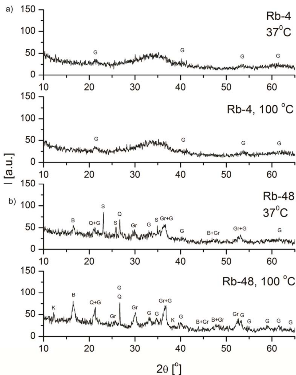
Слика 6.16: Резултати дифракционе анализе талога из дренава бунара Rb-4 и Rb-48 са београдског изворишта, Легенда: G–Гетит ( \alpha -FeOOH), Q–Кварц ( \text{SiO}_2 ), Gr–Греигеит ( \text{Fe}_3\text{S}_4 ), S–моноклинични сумпор ( \text{S}_8 ), B–Берналит \text{Fe}(\text{OH})_3 , K–Каолинит ( \text{Al}_2\text{Si}_2\text{O}_5(\text{OH})_4 )
