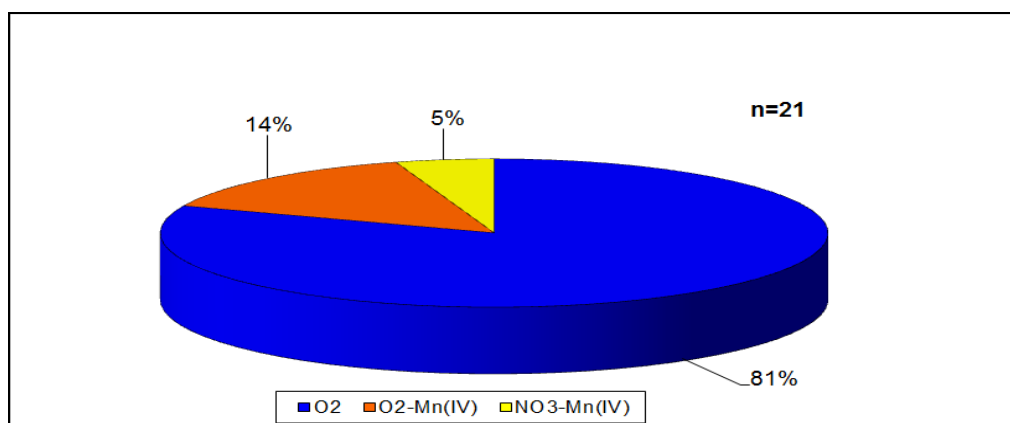
Слика 5.6: Процентуални удео преовлађујућих редокс – реакција у узетим узорцима подземних вода из бунара и пијезометара са изворишта Трновче
