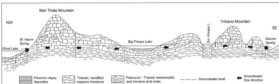
Сл. 3. Хидрогеолошки профил а-а` (АМАТАЈ et al. 2005) Fig. 3. Hydrogeological cross-section a-a` (АМАТАЈ et al. 2005)
