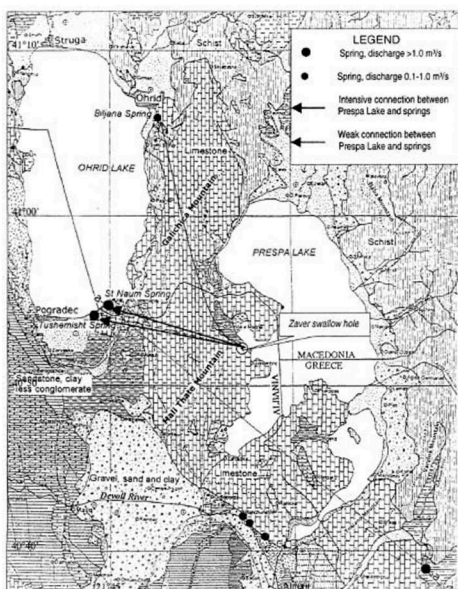
Сл. 2. Шематска хидрогеолошка карта шире околине Охридског и Преспанског језера (AMATAJ et al. 2005)
