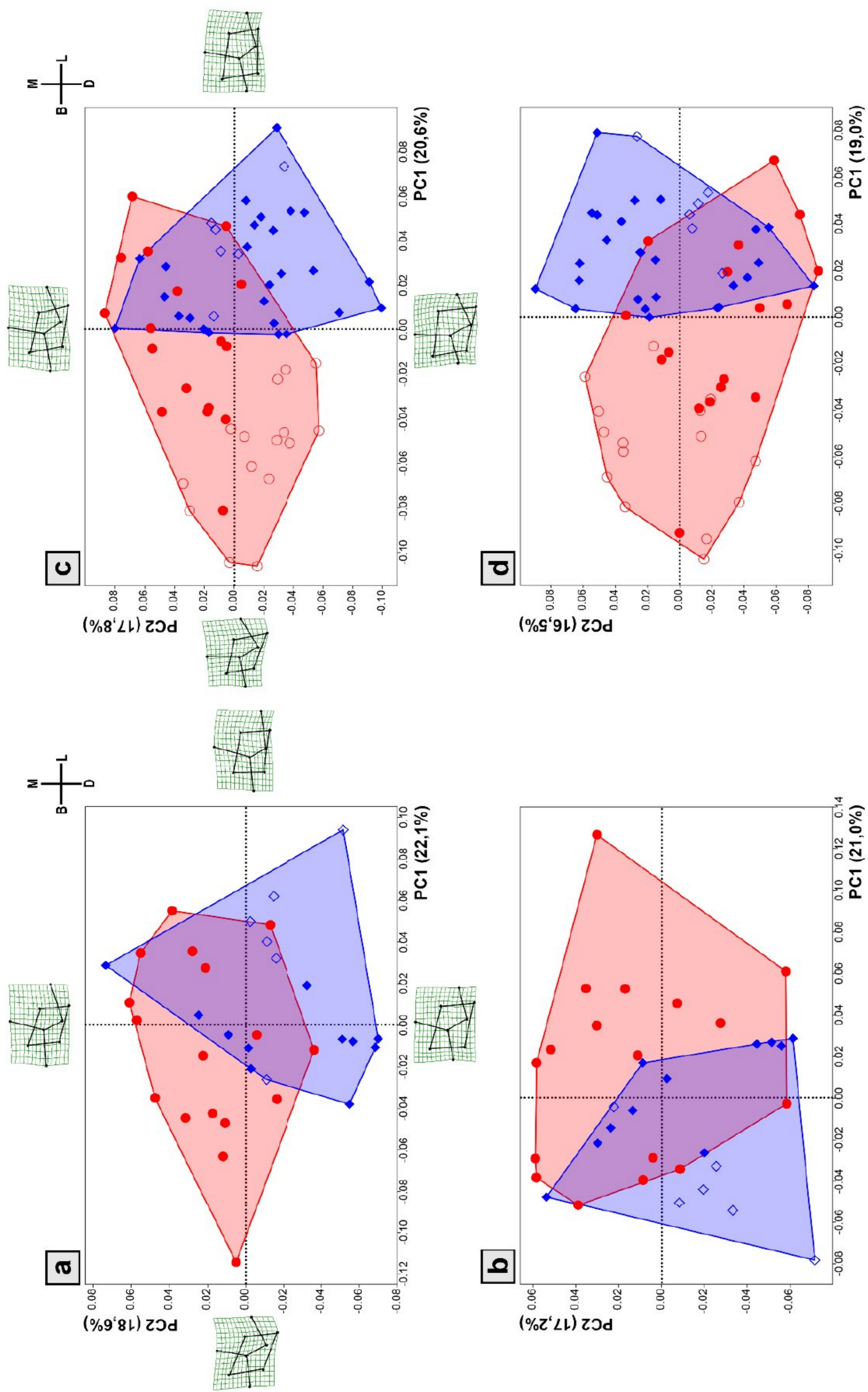
Slika P7. Projekcije pojedinačnih primeraka M1 na prve dve glavne komponente (PC1 i PC2) u prostoru oblika i forme za model Spec2 na manjem ( n = 34 ; a, b) i većem ( n = 64 ; c, d) uzorku. Za dodatna pojašnjenja pogledati Sliku P6 .
