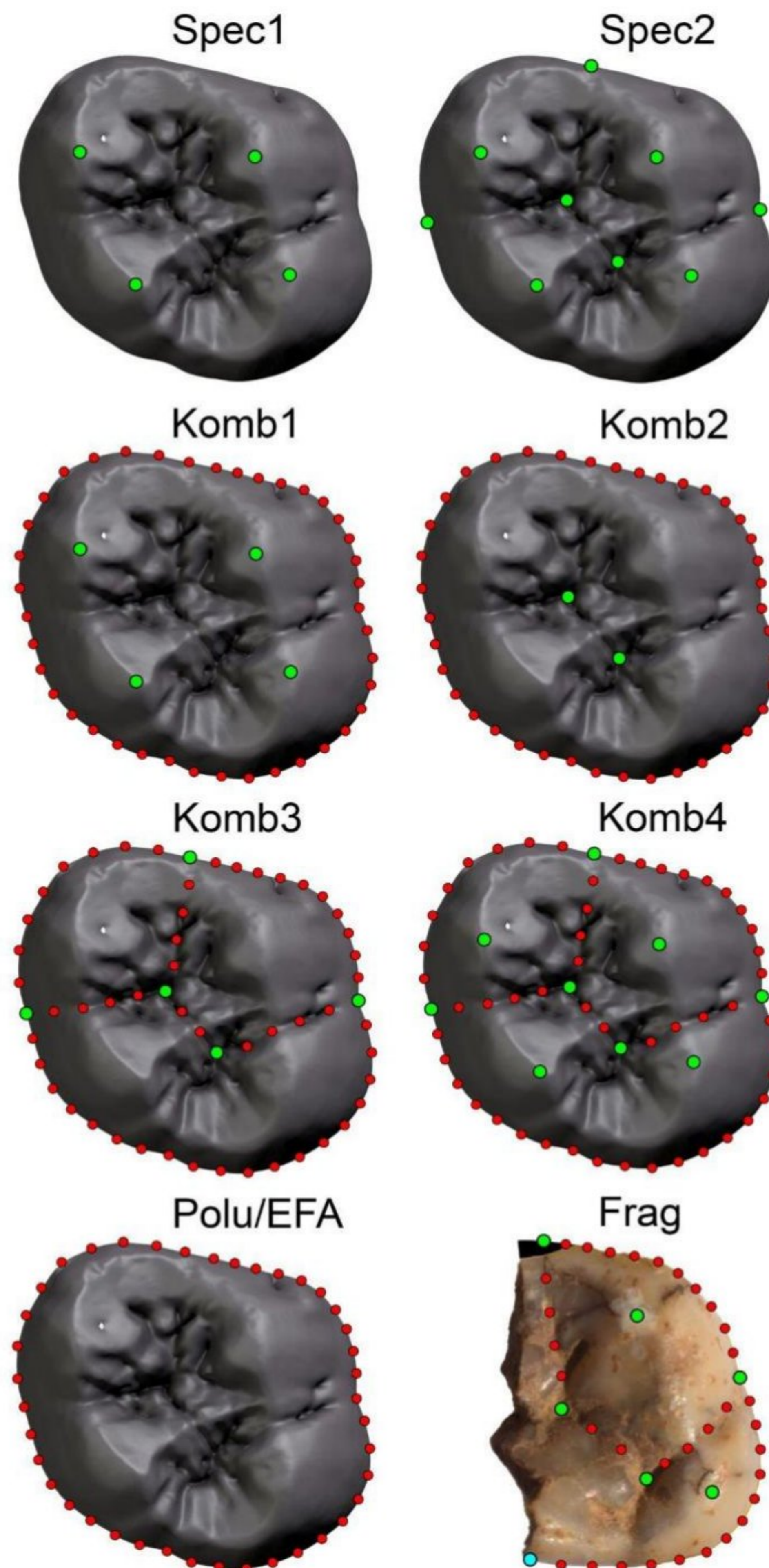
Slika 16. Konfiguracije specifičnih tačaka (zelene) i polutačaka (crvene) testiranih geometrijskih modela. Pozicioniranje dopunske specifične tačke (svetloplava) za konfiguraciju „Frag” je pojašnjeno na Slici P3 . Okluzalna projekcija 3D modela molara (fosilni M1 dex. primerak LQH18) kreirana je u Blender 2.79 okruženju, a sama ilustracija u programu Adobe Photoshop CS6.
