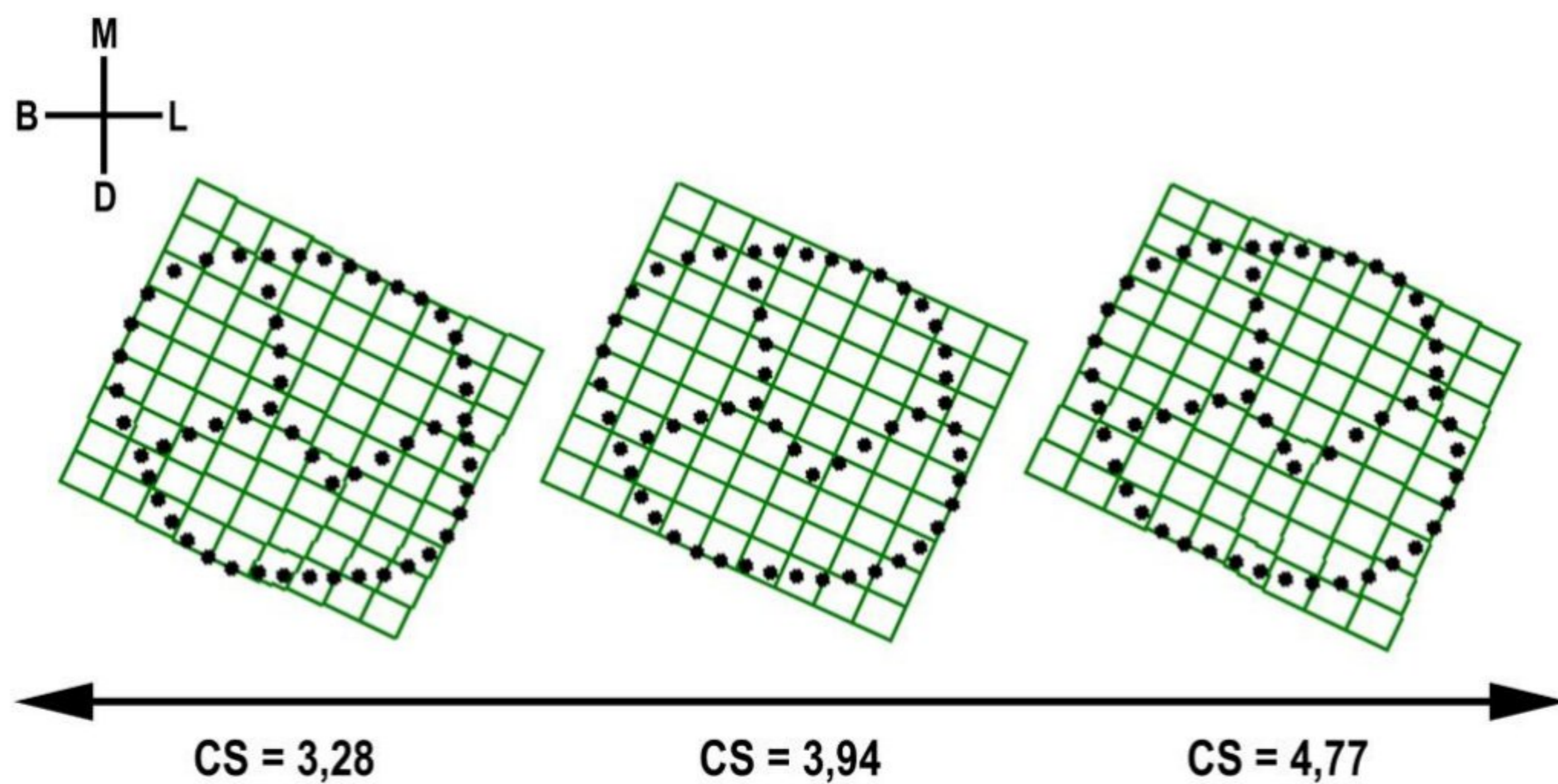
Slika 26. Alometrijske promene oblika krunice M1 za model Komb3A na potpunom uzorku ( n = 80 ), zasnovane na multivarijantnoj regresiji varijabli oblika na prirodni logaritam veličine centroida ( \ln CS ). TPS deformacije mreže ilustruju morfološke varijante povezane sa promenom vrednosti veličine centroida (CS). Prikazana je transformacija oblika od srednje vrednosti CS (centralna slika) ka minimalnoj (levo) i maksimalnoj (desno) veličini. Orijehtacija krunice: B = bukalno, L = lingvalno, M = mezijalno, D = distalno. Deformacione mreže su kreirane u programu tpsRegr, dok je sama ilustracija sačinjena u programu Adobe Photoshop CS6.
