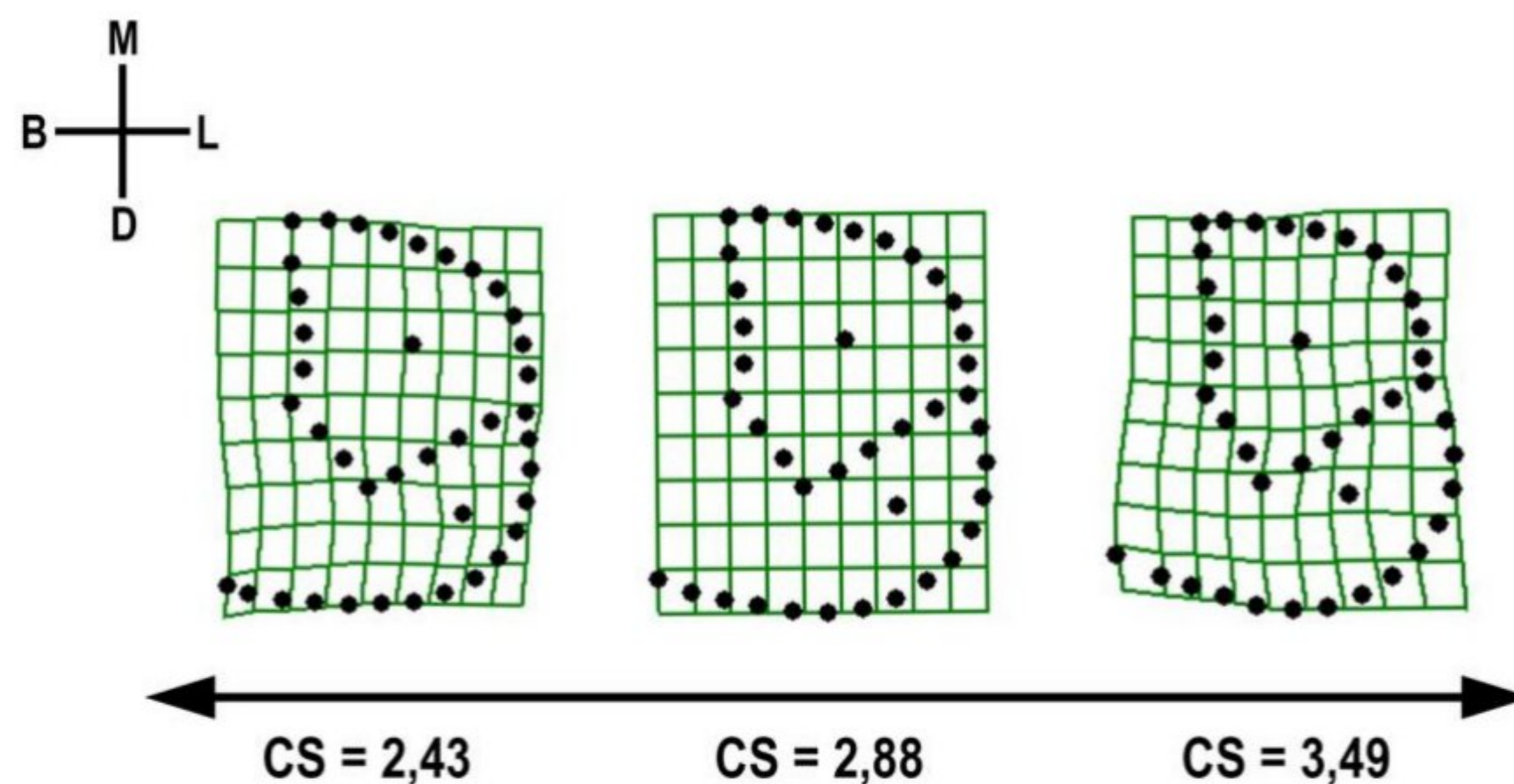
Slika 27. Alometrijske promene oblika krunice M1 za model FragA na potpunom uzorku ( n = 79 ). Prikazana je transformacija oblika od srednje vrednosti CS (centralna slika) ka minimalnoj (levo) i maksimalnoj (desno). B = bukalno, L = lingvalno, M = mezijalno, D = distalno. Deformacione mreže su kreirane u programu tpsRegr, dok je sama ilustracija sačinjena u Adobe Photoshop CS6 okruženju.
