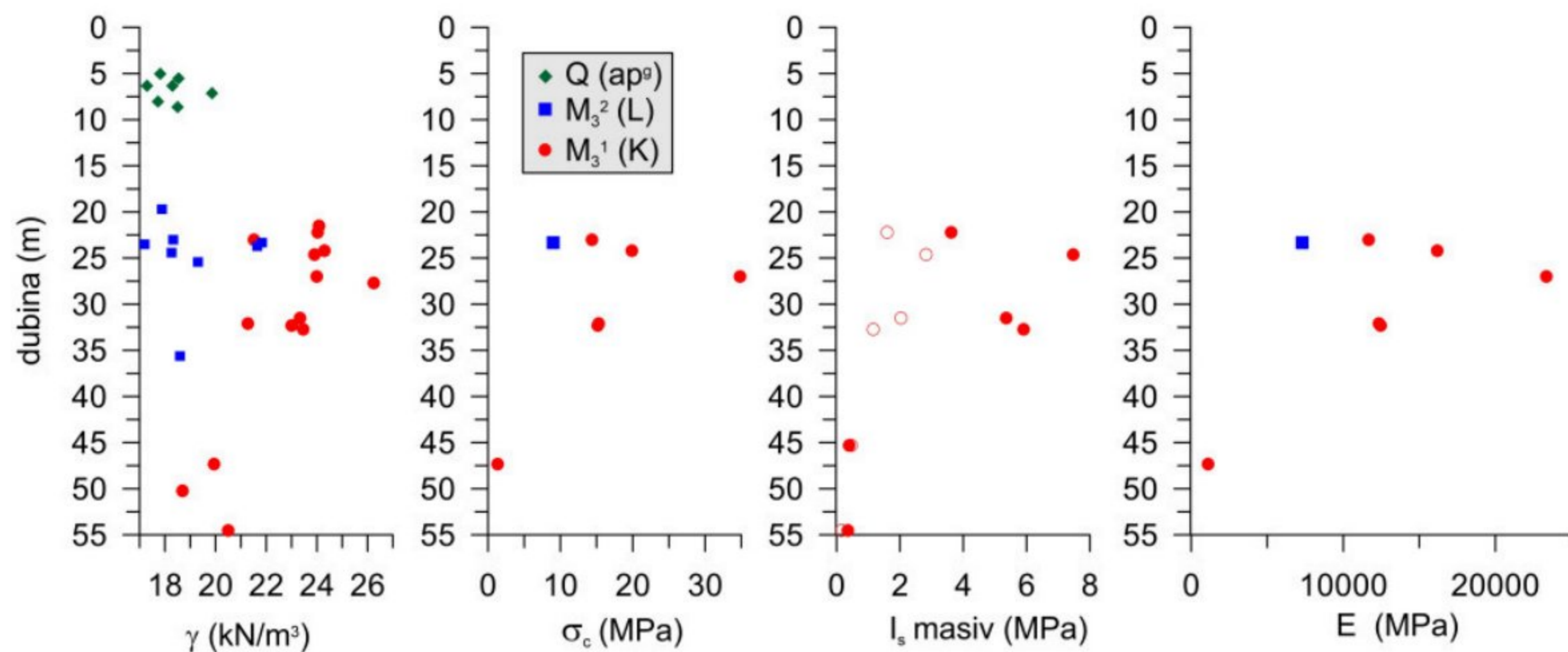
Slika 4. Prikaz pojedinih parametara tla i stenskih masa dobijen laboratorijskim ispitivanjima
