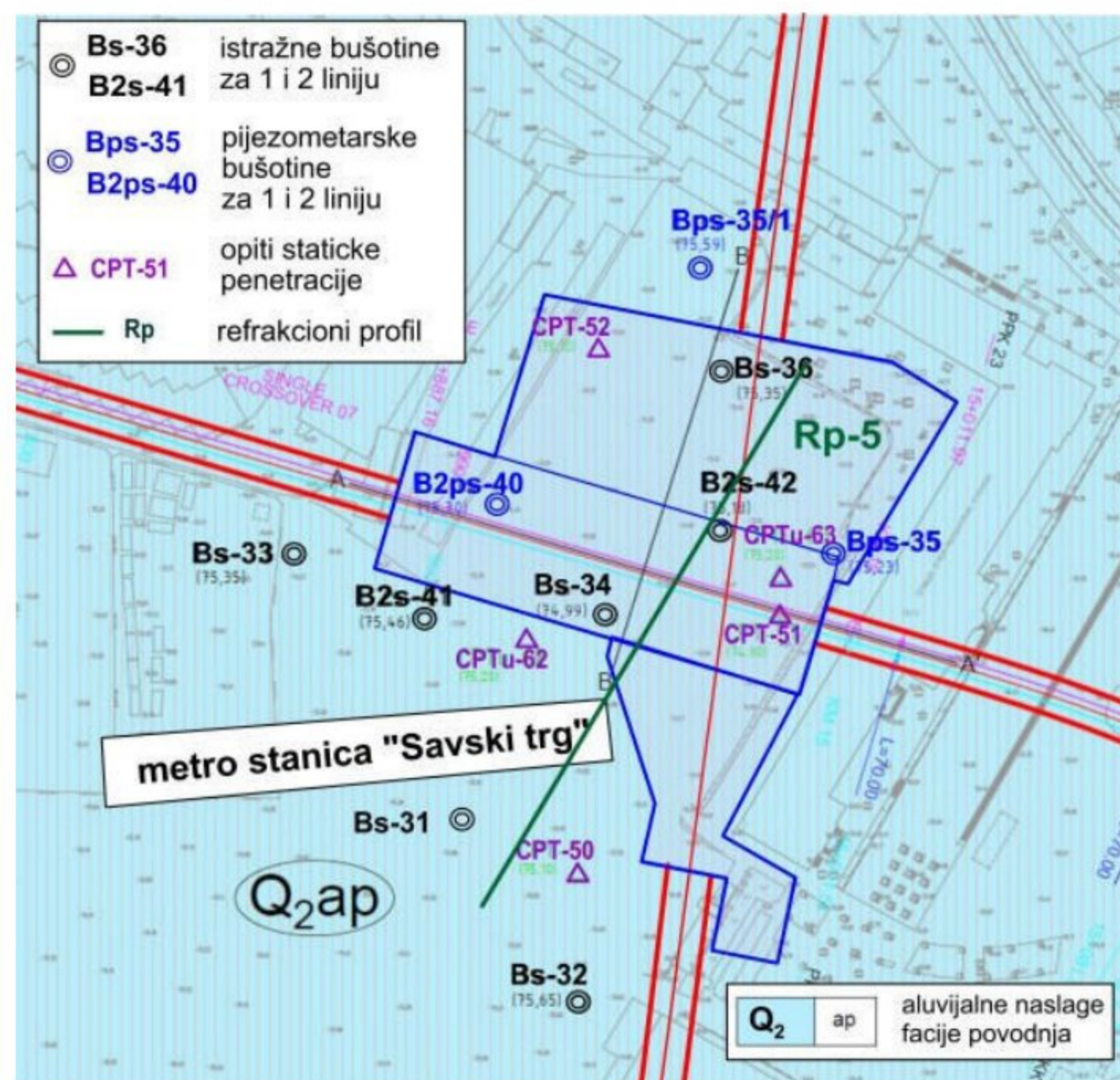
Slika 2. Inženjerskogeološka karta sa rasporedom istražnih radova
