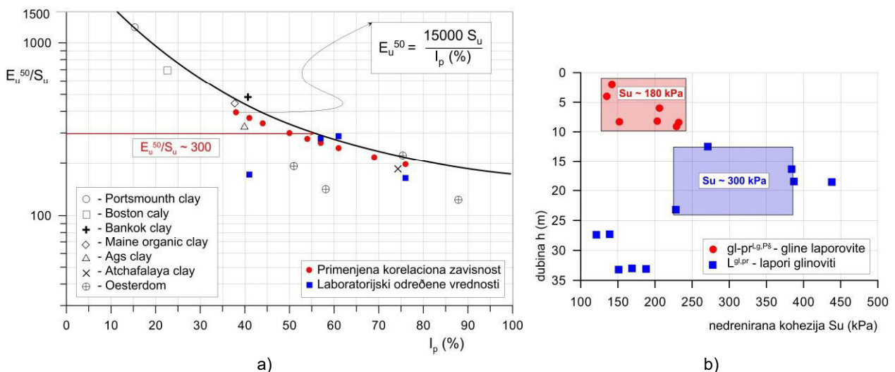
Slika 6. Karakteristične vrednosti nedrenirane čvrstoće smicanja i nedreniranog modula elastičnosti
