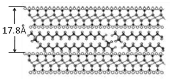
Slika 64. Model slaganja HDTMA + katjona u vidu lateralnog dvosloja (Zhu et al., 2003)
