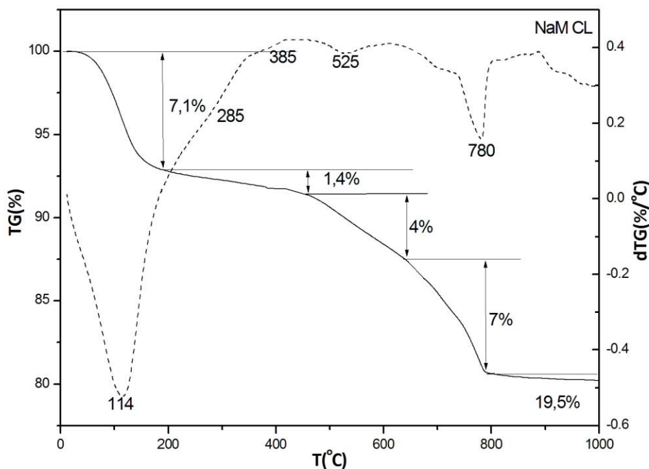
Slika 42. TG i DTG krive Na-montmorionita sa klomazonomom
