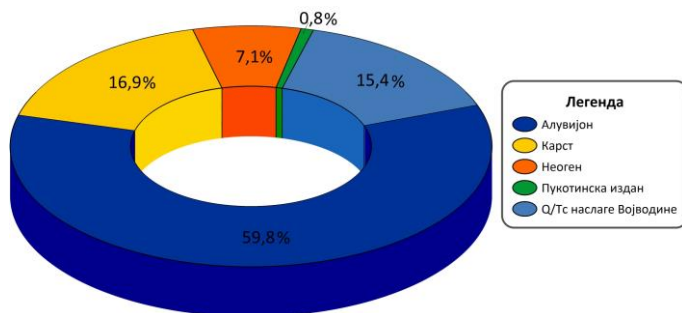
Слика 2. Процентуална заступљеност типова издани у водоснабдевању становништва Србије подземним водама (према подацима STEVANOVIĆ & DOKMANOVIĆ, 2015) Fig. 2. Participation of aquifer types (in percent) in the water supply of the population of Serbia with groundwater (after STEVANOVIĆ & DOKMANOVIĆ, 2015)
