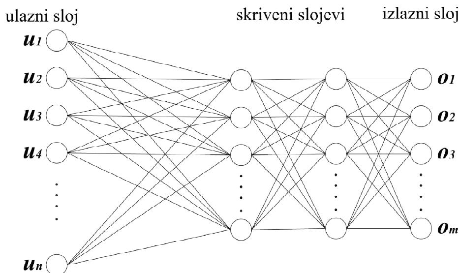
Slika 4.11 – Višeslojna arhitektura mreže
