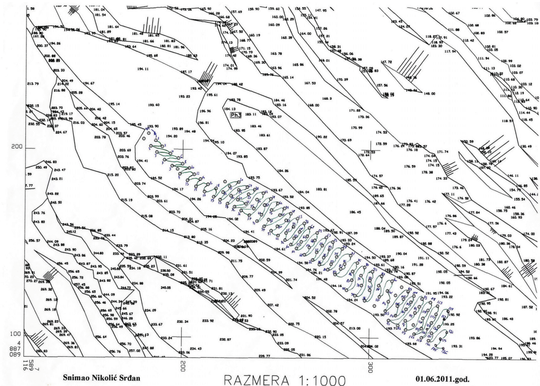
Slika 5.1 – Geodetski snimak minske serije iz dnevnika miniranja
