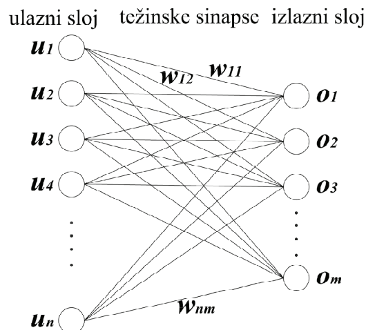
Slika 4.10 – Jednoslojna arhitektura mreže
